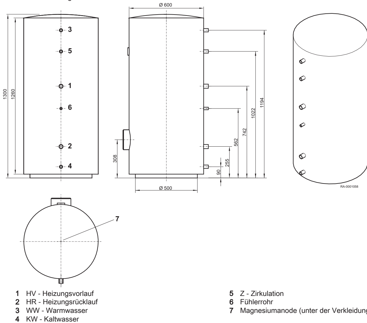
Abb.1 Abmessungen und Anschlüsse
