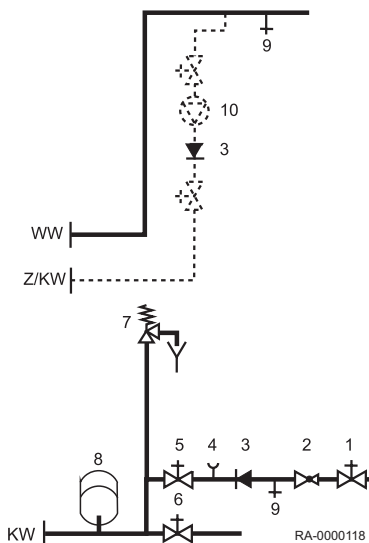
Abb.2 Kaltwasseranschluss nach DIN 1988
