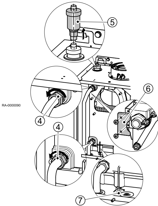
Abb.41 Wärmetauscher ausbauen
