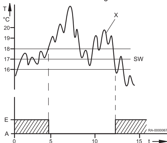
Abb.25 Sommer-/Winterheizgrenze
