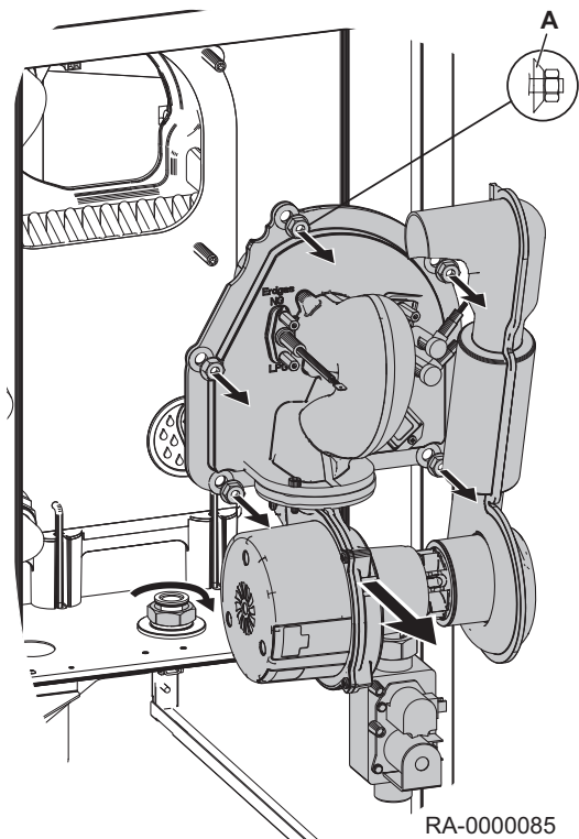
Abb.40 Gasbrenner ausbauen
