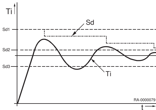
Abb.33 Schaltdifferenz
