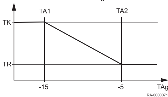
Abb.29 Reduziert-Anhebung
