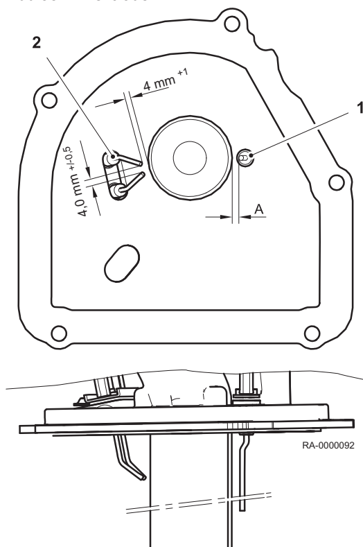
Abb.38 Elektroden
