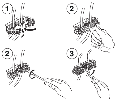
Abb. 19 Zugentlastungen
