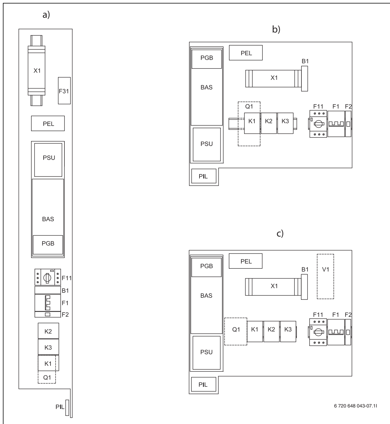
Bild 33 Übersicht Leiterplatte
