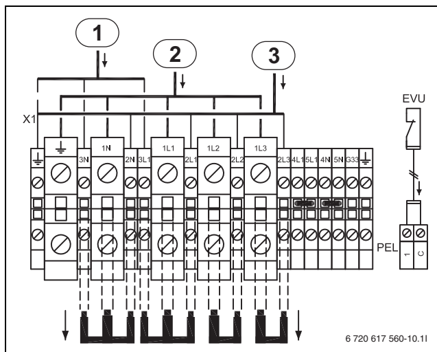
Bild 44 Alternative B, WPS 13-1 - 17-1
