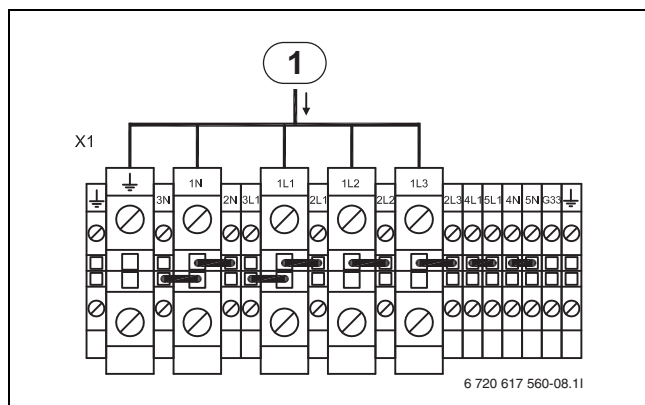
Bild 42 Standardausführung, WPS 13-1 - 17-1
