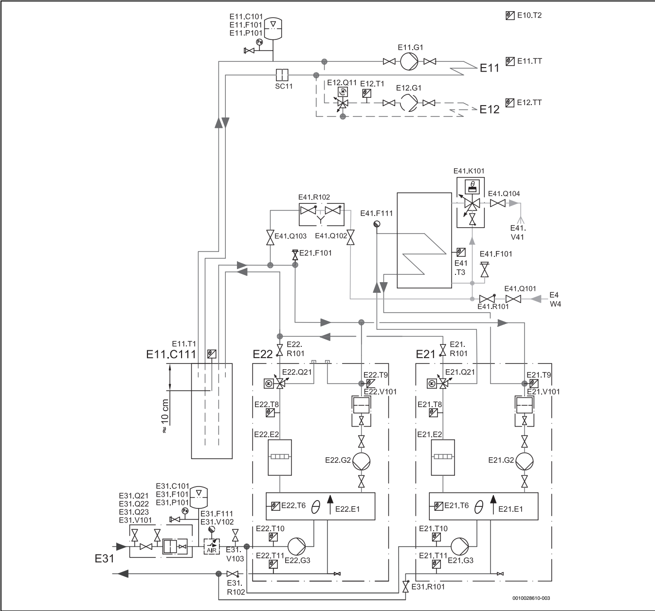
Bild 72 Zwei Wärmepumpen (Kaskadenschaltung) mit gemischtem und ungemischtem Heizkreis, Pufferspeicher und externem Warmwasserspeicher.
