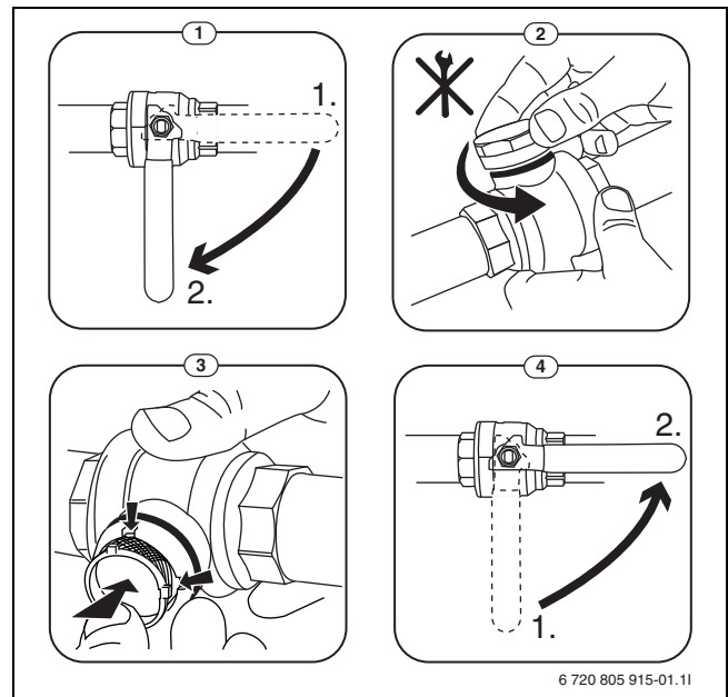
Bild 71 Filtervariante ohne Sicherungsring
