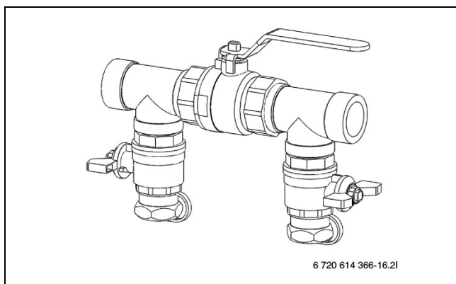
Bild 22 Befülleinrichtung WPS 13-1...17-1
