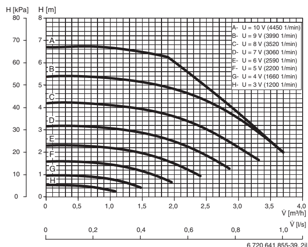
Heizungspumpe primär 10-1 - 13-1
