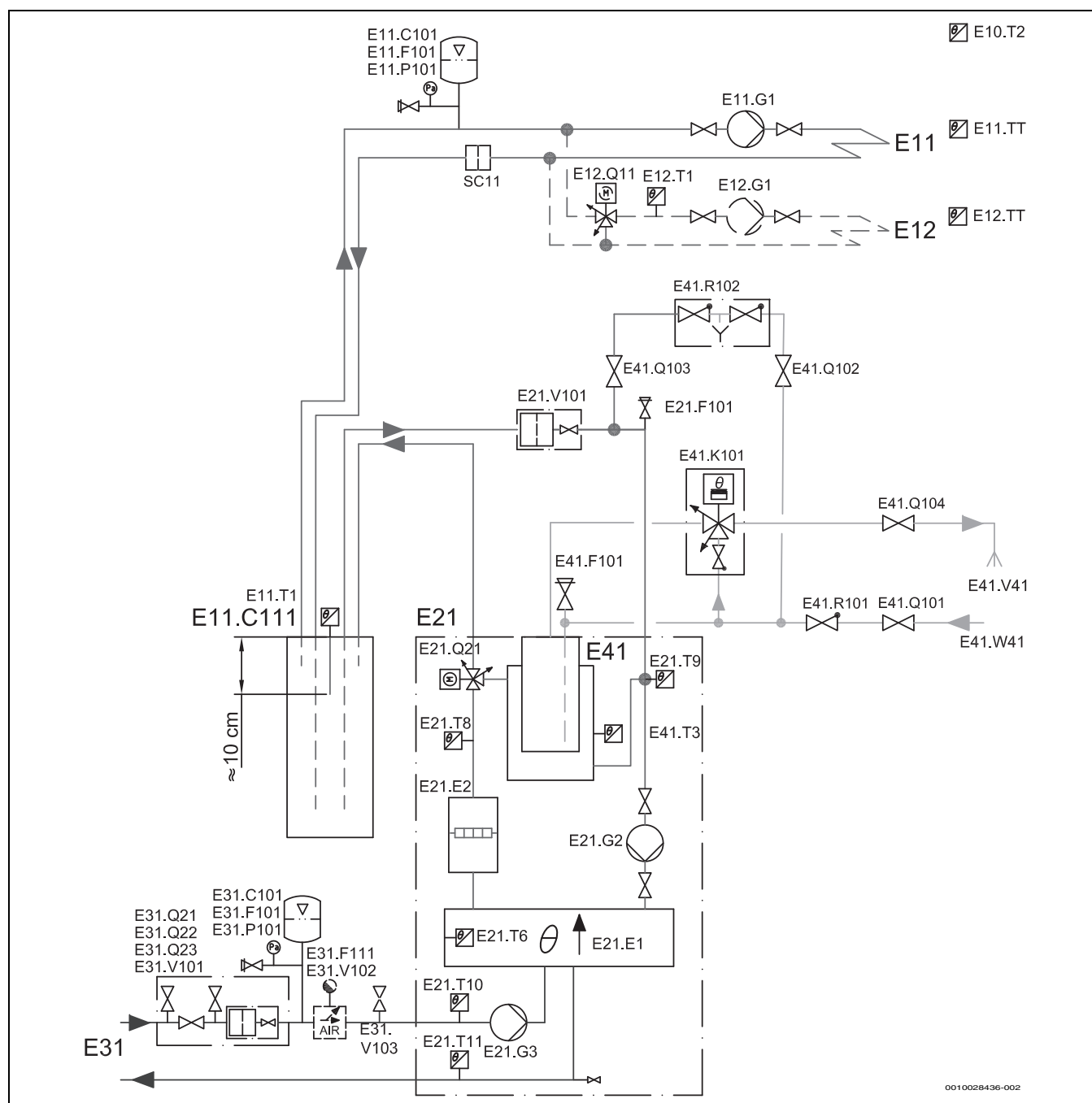
Bild 10 Monoenergetisch, ungemischter Heizkreis mit Pufferspeicher
