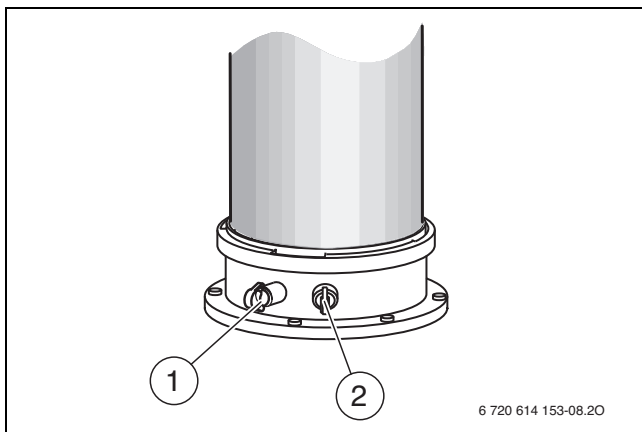
Bild 114 Abgasmessstutzen und Verbrennungsluft-Messstutzen
