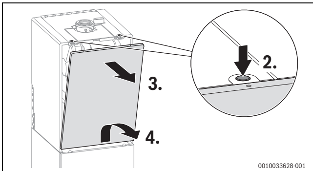
Bild 118 Vorderteil der Geräteverkleidung abnehmen
