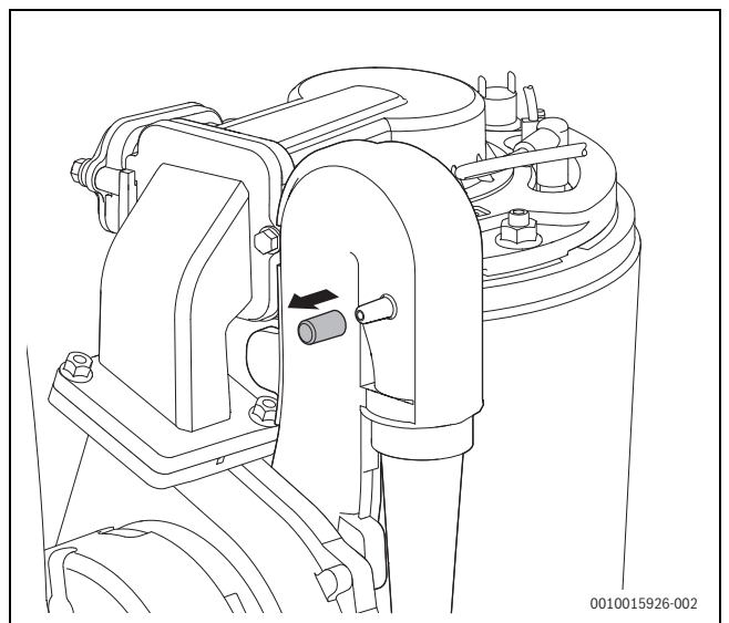
Bild 121 Messstutzen an der Mischeinrichtung
