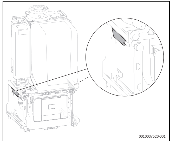
Bild 61 Gerät an den grau hervorgehobenen Stellen anheben und zum Speicher transportieren
