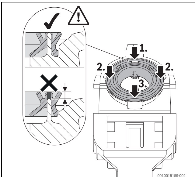
Bild 155 Dichtung andrücken
