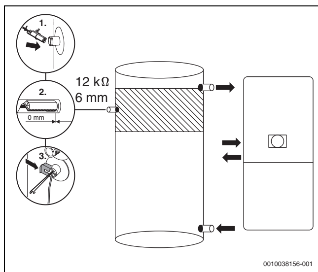
Bild 78 Pufferspeicher-Temperaturfühler einsetzen
