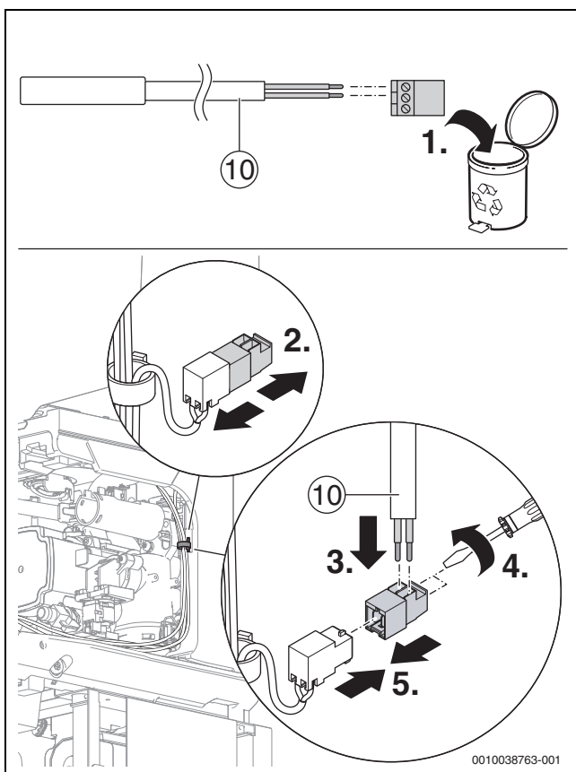
Bild 93 Pufferspeicher-Temperaturfühler anschließen
