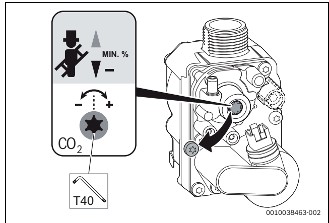
Bild 113 CO 2 /O 2 -Gehalt bei minimaler Nennwärmeleistung einstellen
