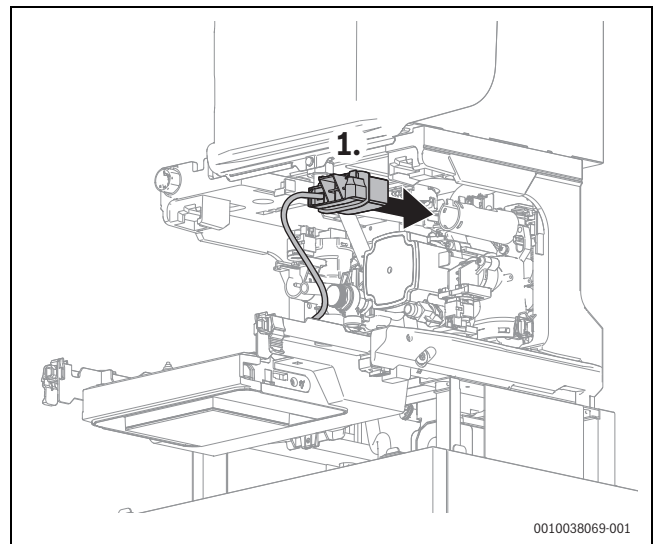
Bild 69 Funkmodul-Halter auf die Rückseite des Geräts führen
