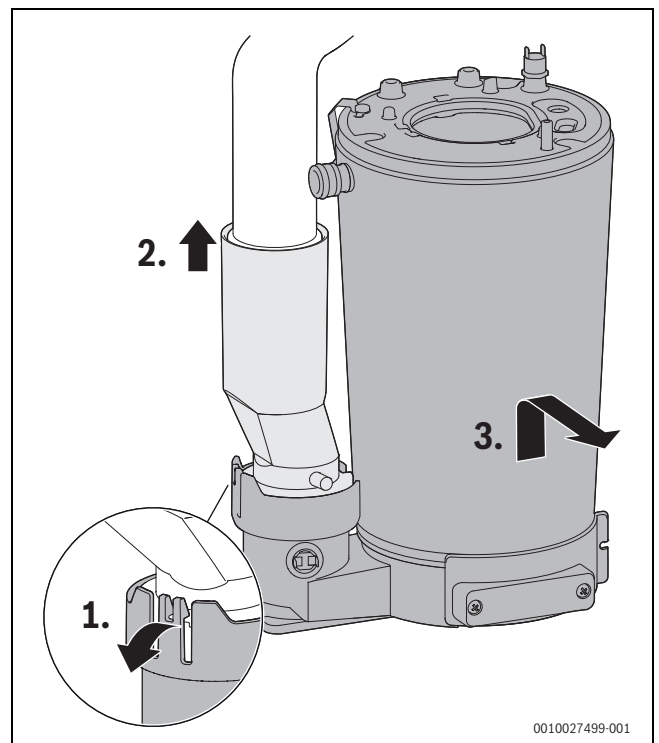
Bild 139 Wärmeblock ausbauen
