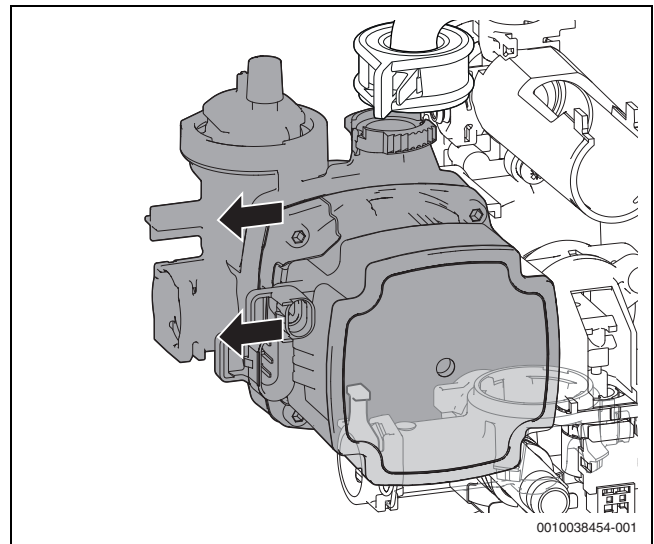
Bild 143 Heizungspumpe aus dem Gerät nehmen
