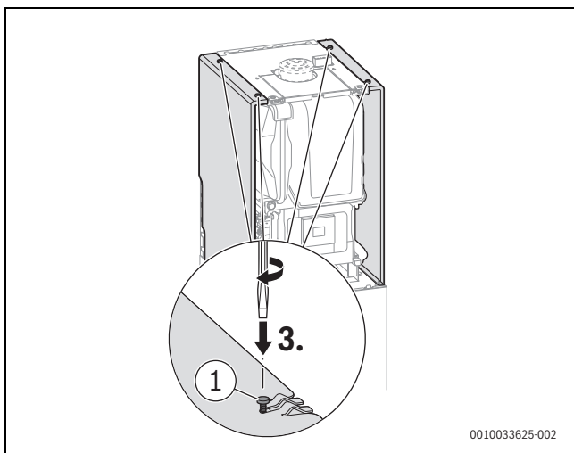
Bild 97 Seitenteile der Geräteverkleidung befestigen
