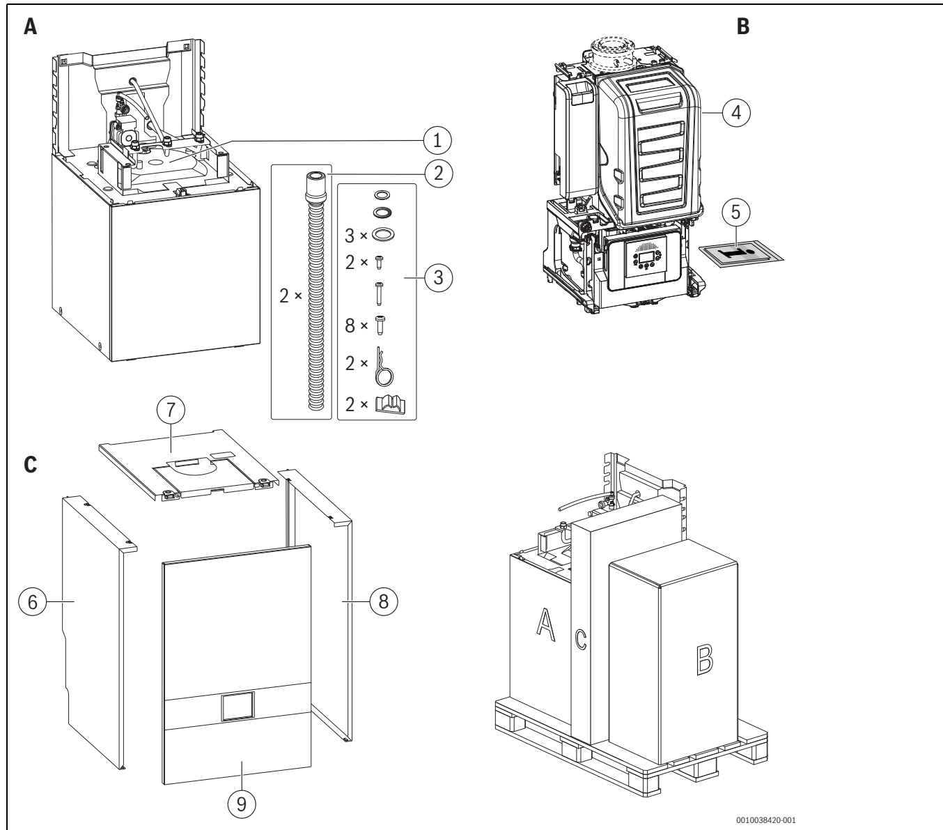
Bild 3 Lieferumfang
