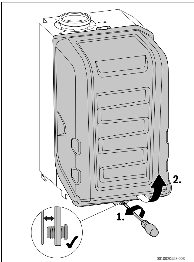
Bild 119 Brennerhaube abnehmen
