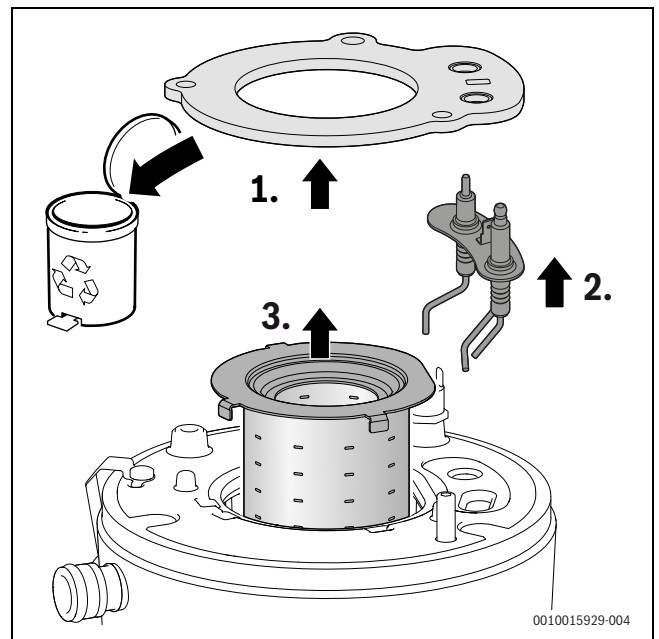
Bild 129 Brenner herausnehmen
