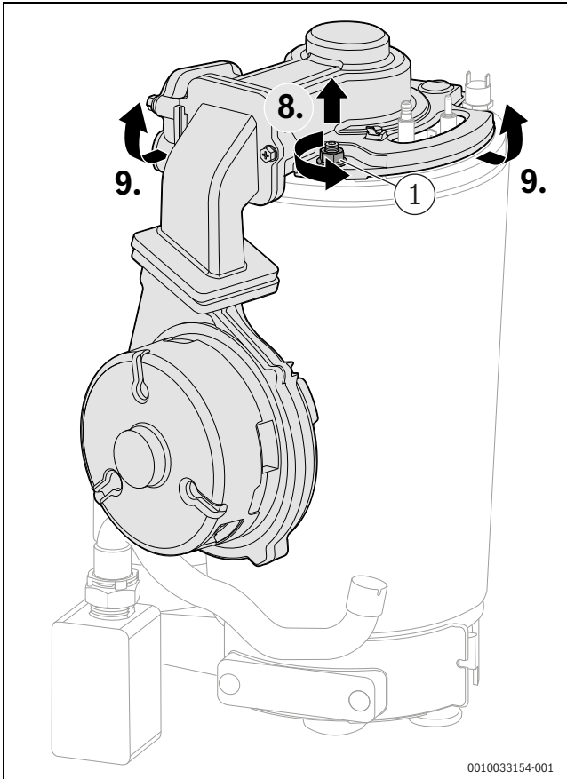
Bild 126 Brennerdeckel mit Gebläse und Mischeinrichtung abnehmen
