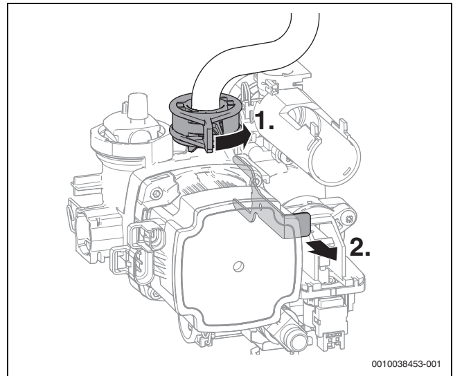
Bild 142 Heizungspumpe entriegeln
