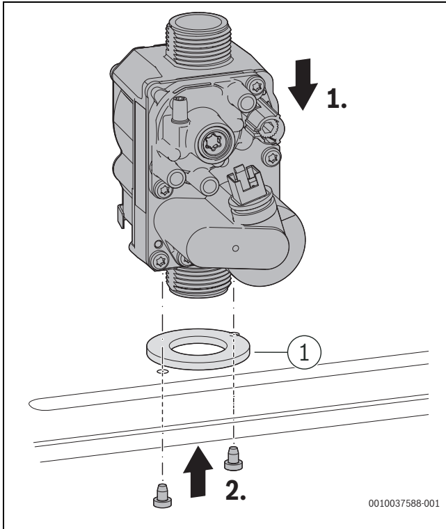
Bild 148 Gasarmatur einbauen
