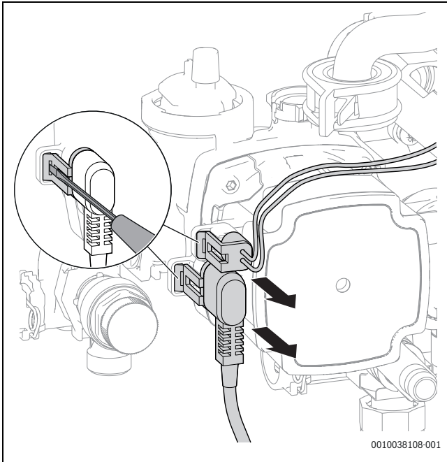
Bild 140 Stecker an der Heizungspumpe abziehen
