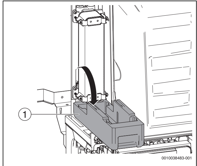
Bild 157 Hartschale als Auffangbehälter verwenden
