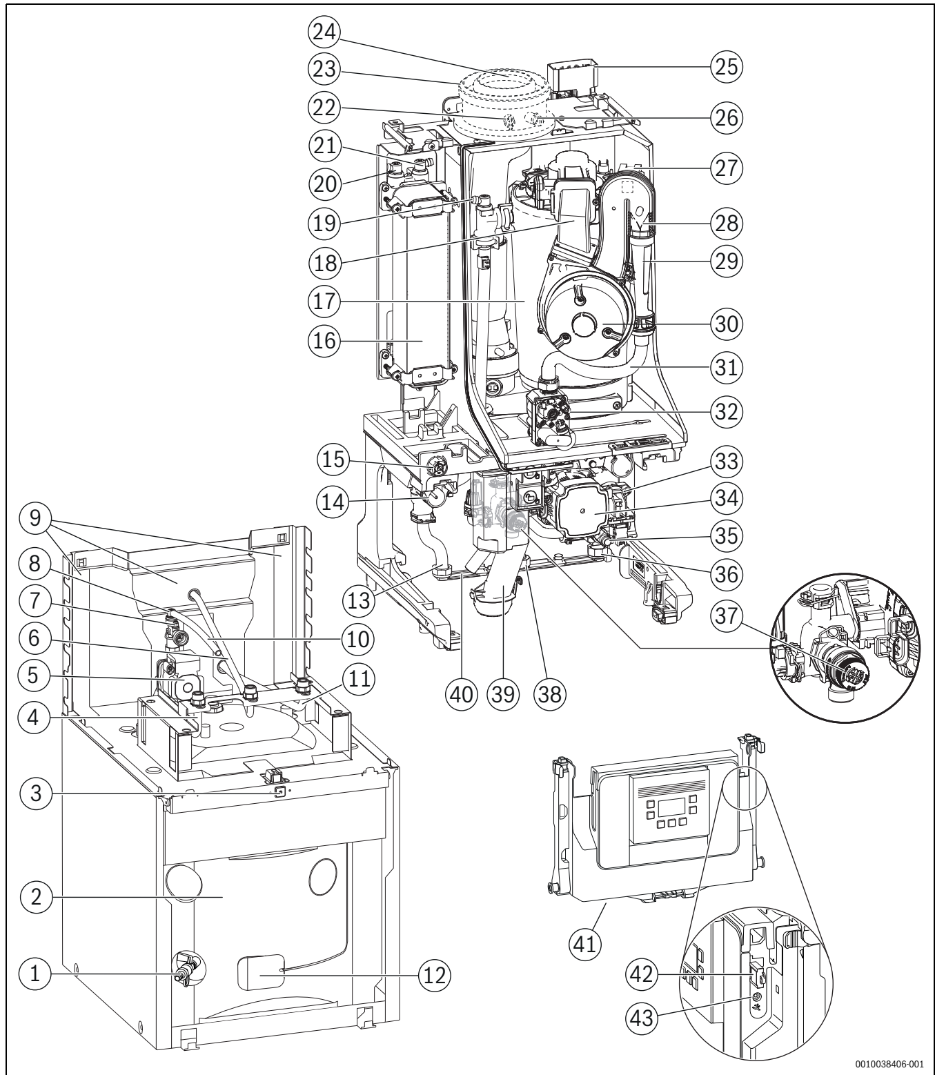
Bild 4 Gerät und Warmwasserspeicher
