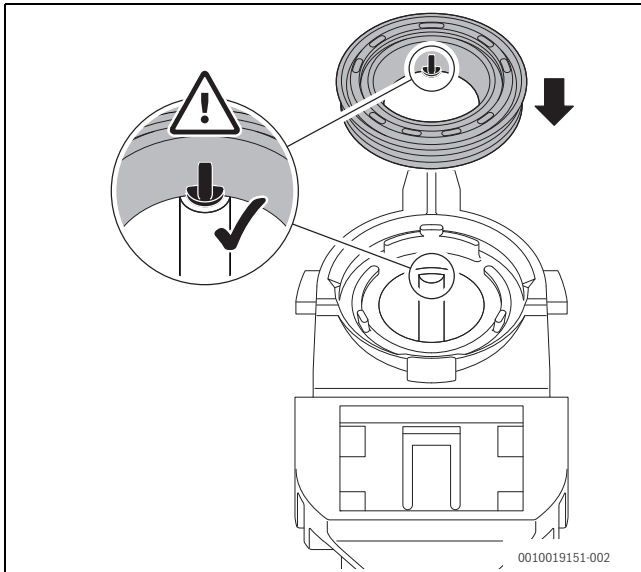
Bild 154 Neue Dichtung am Kondensatsiphon ausrichten
