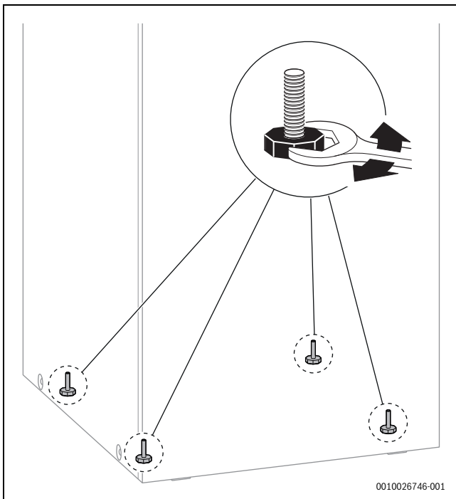
Bild 102 Am endgültigen Aufstellort Unebenheiten des Fußbodens mit den Stellfüßen ausgleichen
