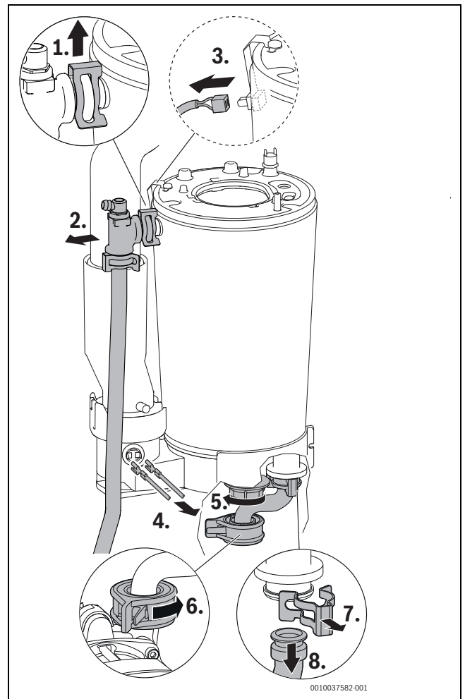
Bild 138 Vorlaufrohr lösen, Kabel abziehen und Rücklaufrohr lösen
