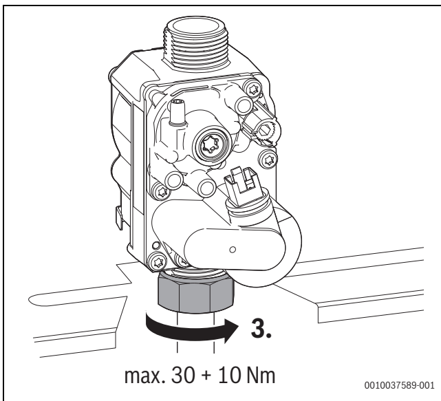
Bild 149 Anzugsdrehmoment beachten
