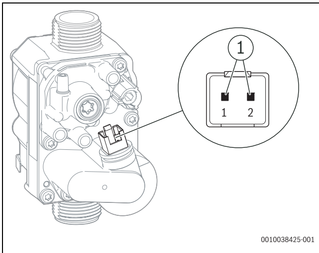
Bild 122 Messstellen an der Gasarmatur
