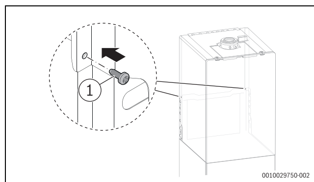
Bild 100 Seitenteile der Geräteverkleidung auf der linken und rechten Seite festschrauben
