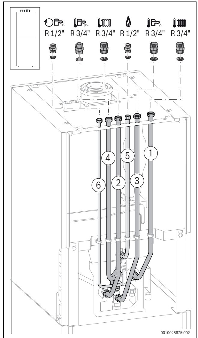
Bild 57 Zubehör CS 33 montiert
