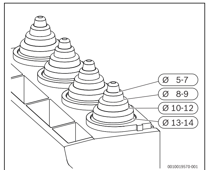
Bild 89 Zugentlastung an Kabeldurchmesser anpassen
