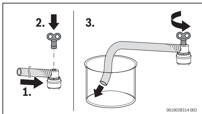
Bild 81 Warmwasserkreis entlüften
