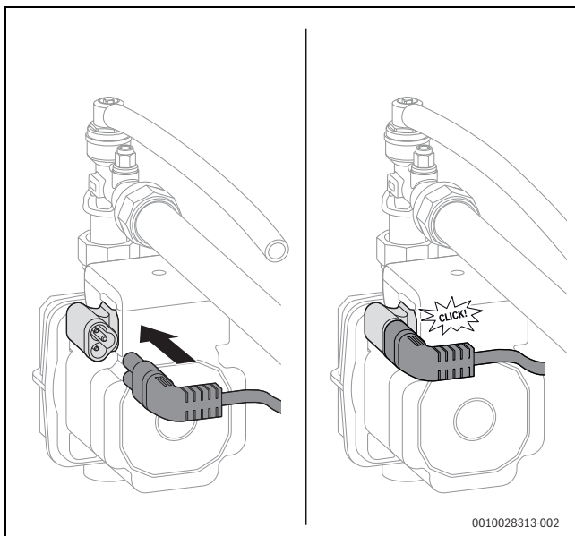
Bild 92 Schichtladepumpe elektrisch anschließen
