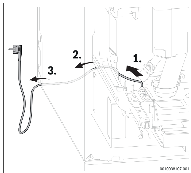
Bild 94 Kabelführung des Netzkabels
