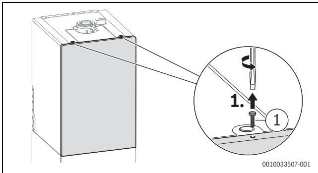
Bild 117 Sicherungsschraube lösen
