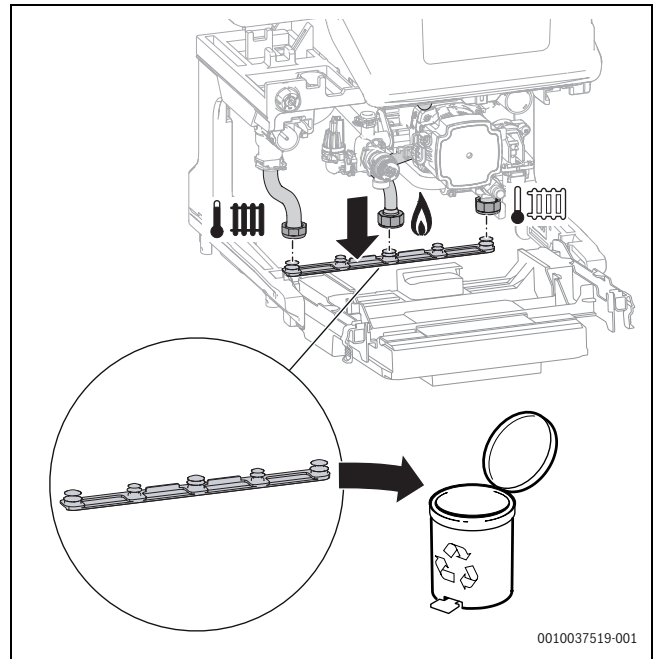
Bild 60 Stopfen am Heizungsanlauf, Gas, Heizungsrücklauf entfernen
