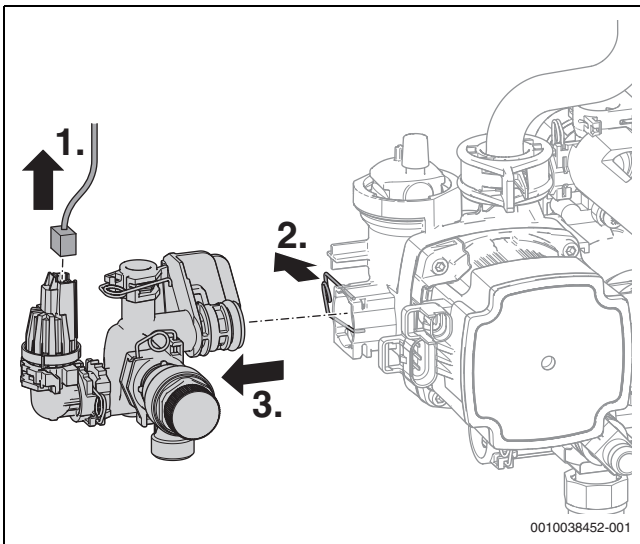
Bild 141 Sicherheitsventil aus dem Gerät nehmen
