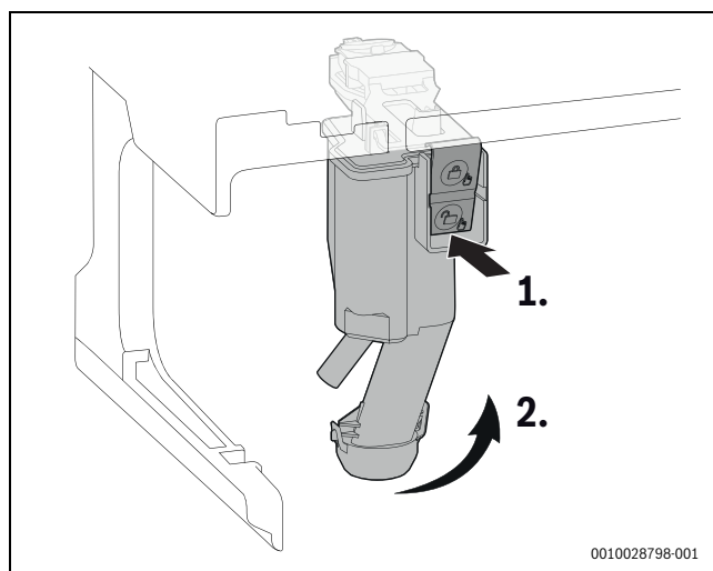
Bild 64 Kondensatsiphon herausnehmen
