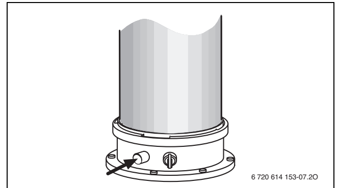
Bild 111 Stopfen abnehmen
