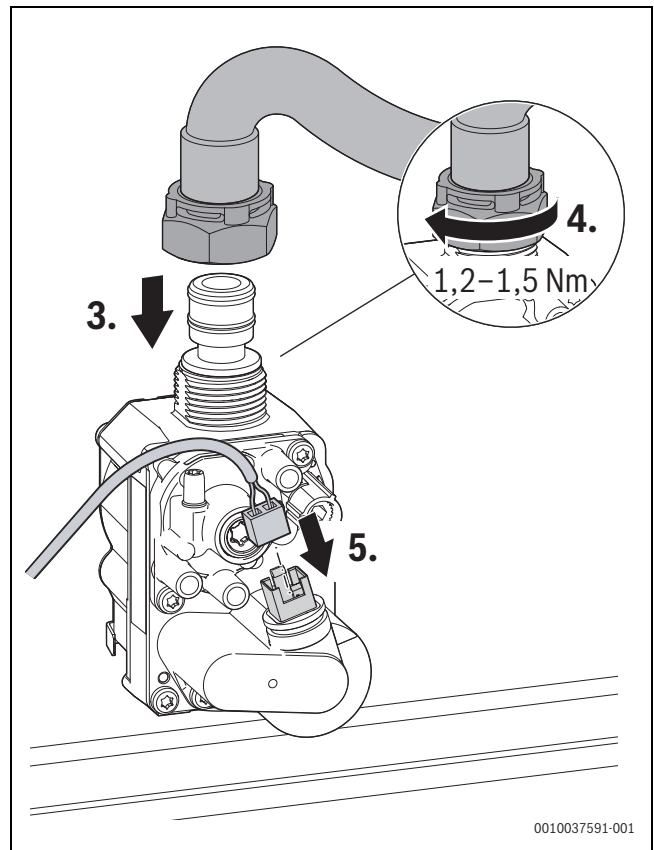
Bild 151 Gasschlauch und Stecker anschließen – Anzugsdrehmoment beachten
