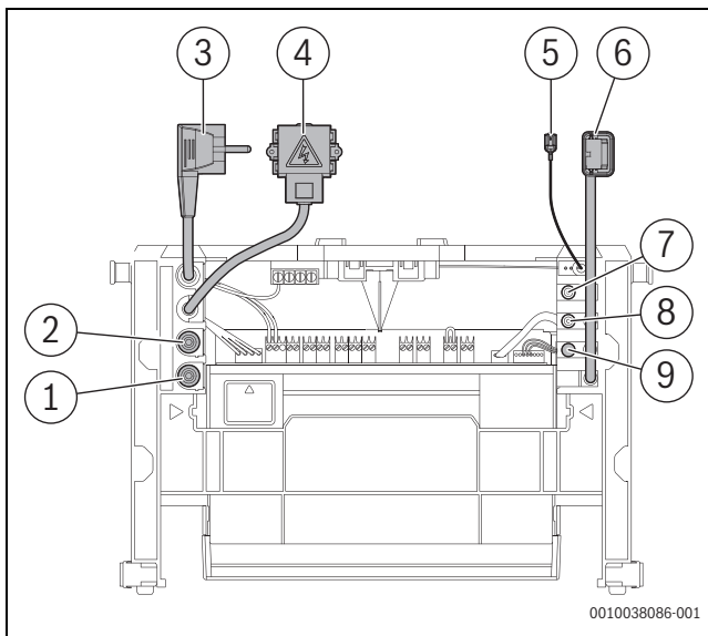
Bild 87 Lieferzustand des Steuergeräts mit angeschlossenen Komponenten
