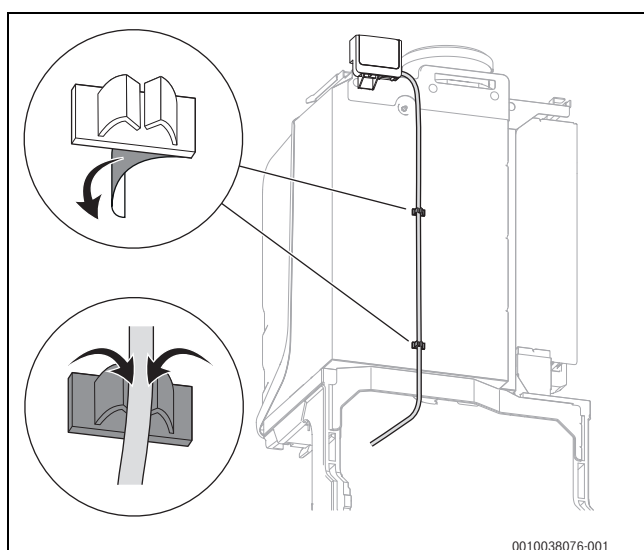
Bild 71 Kabelhalter an der Rückseite des Geräts anbringen und Kabel befestigen
