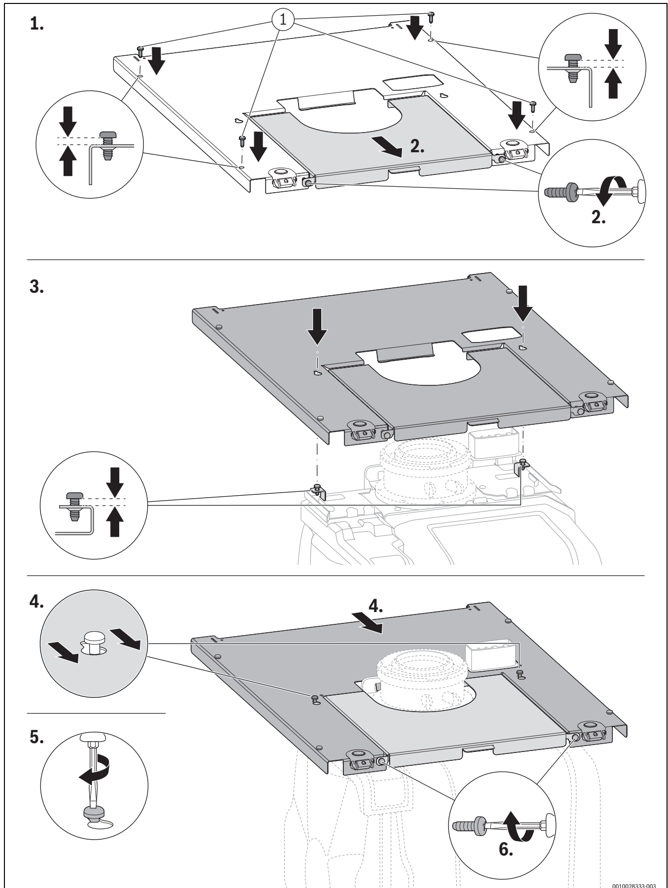
Bild 95 Oberteile der Geräteverkleidung befestigen. Wenn erforderlich können beide Teile der Verkleidung nacheinander eingesetzt werden.
