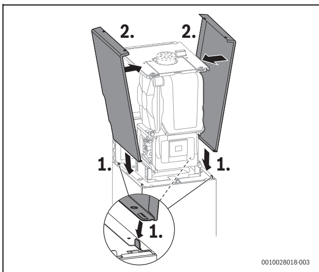
Bild 96 Seitenteile der Geräteverkleidung einsetzen
