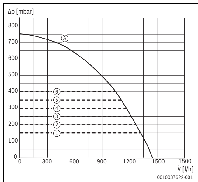
Bild 168 Pumpenkennfelder und Pumpenkennlinie (17/24 kW)
