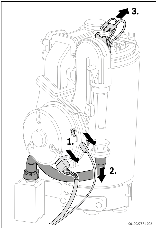
Bild 123 Stecker und Gasschlauch abziehen
