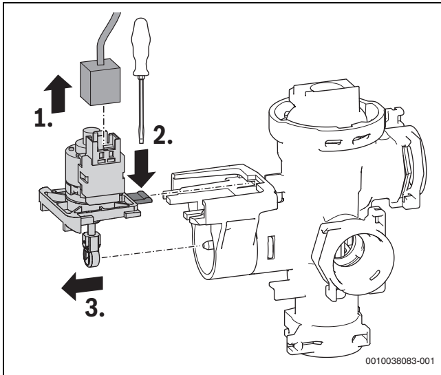
Bild 163 Motor aus dem Gehäuse herausnehmen.
