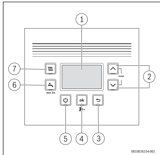
Bild 103 Bedienfeldübersicht
