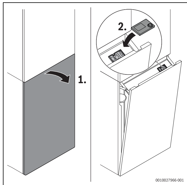
Bild 79 Bedieneinheit Logamatic RC310 einsetzen
