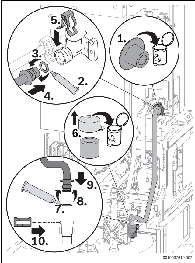
Bild 67 Warmwasserrohr des Speicherladekreises am Speicher anschließen
