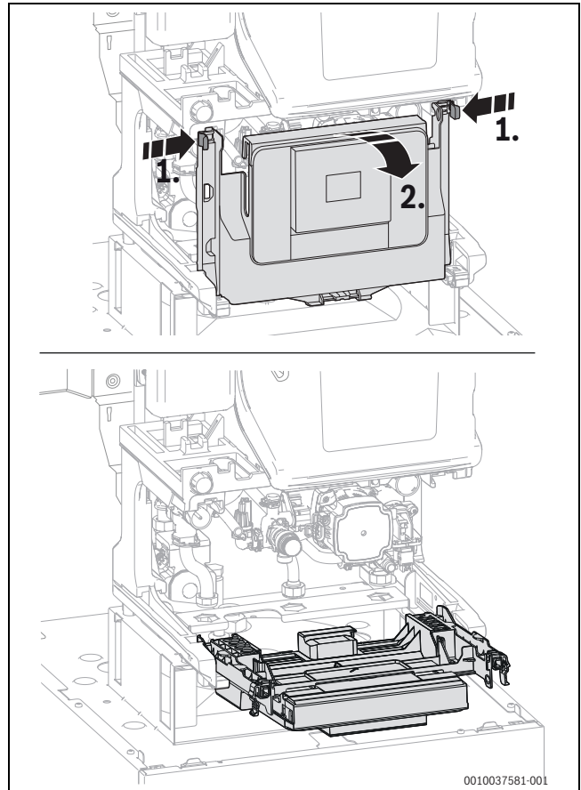
Bild 120 Steuergerät herunterklappen
