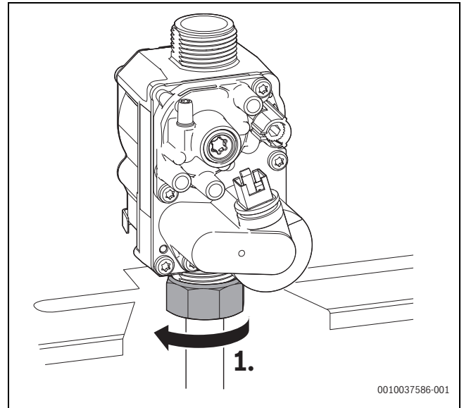
Bild 146 Überwurfmutter lösen
