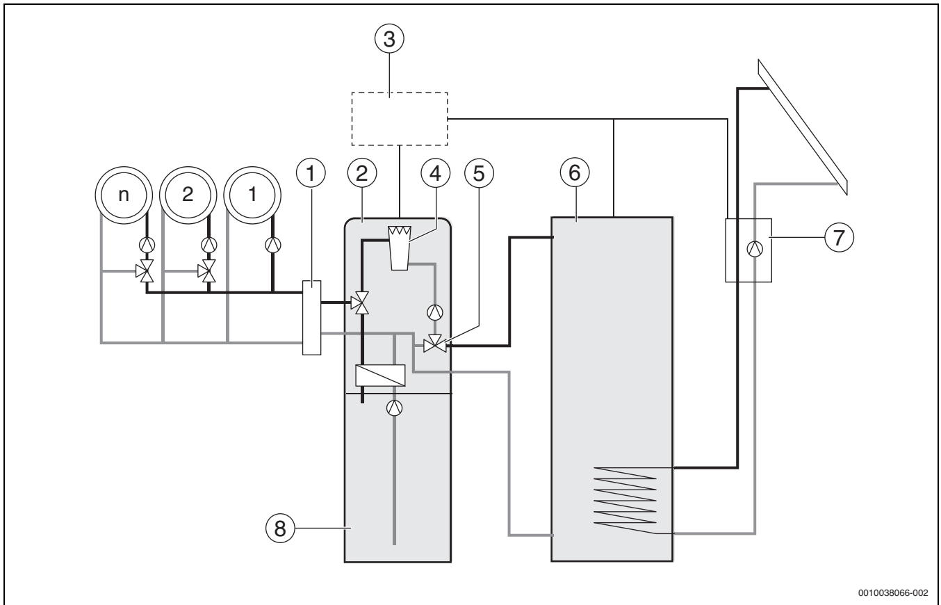
Bild 8 Beispiel: Logamax plus mit Pufferspeicher und Solarthermie
