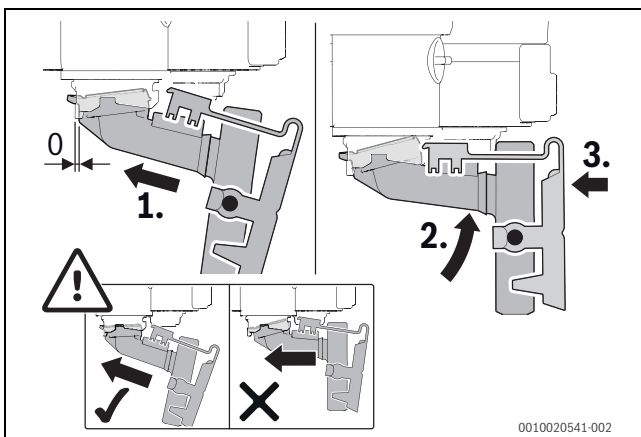
Bild 156 Kondensatsiphon einbauen
