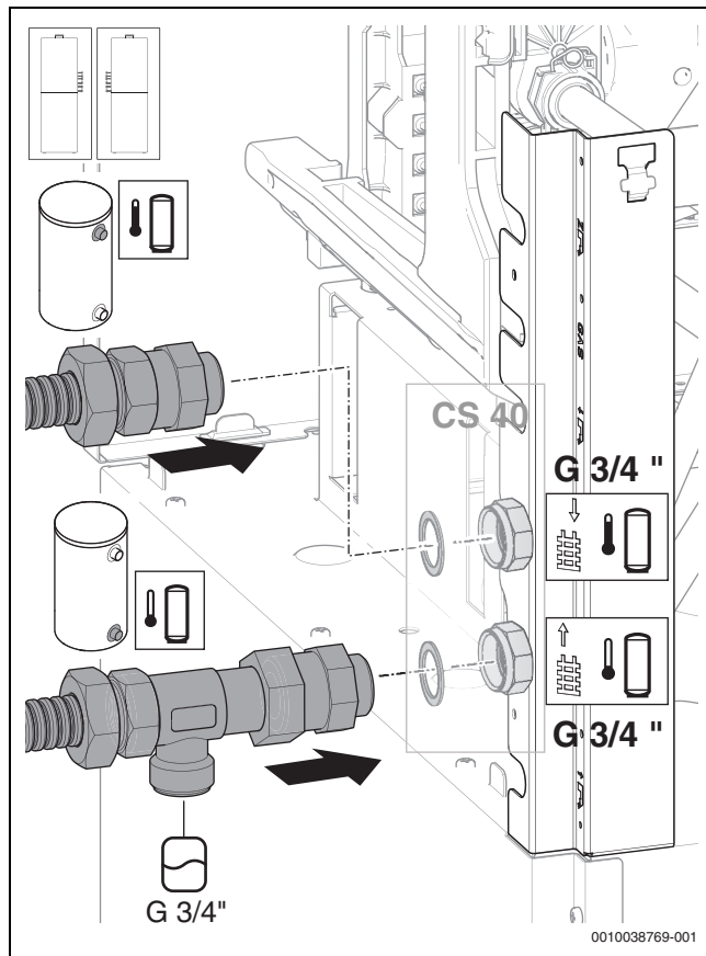
Bild 51 Ausdehnungsgefäß anschließen
