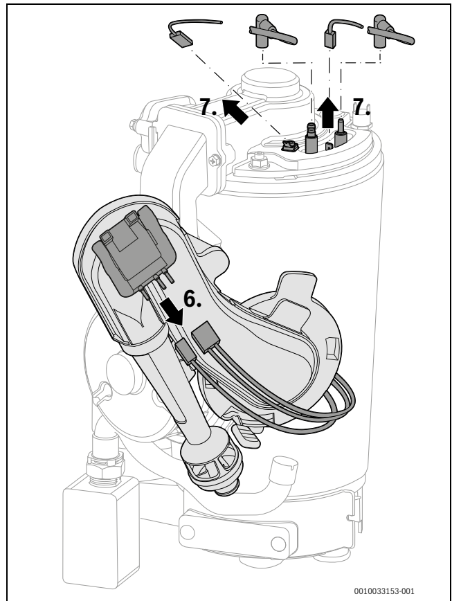
Bild 125 Kabel abziehen
