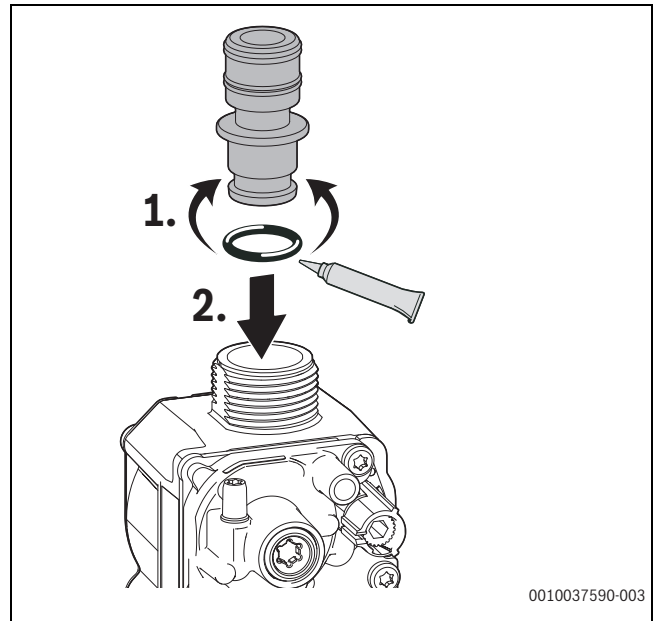
Bild 150 Gasdüse einsetzen
