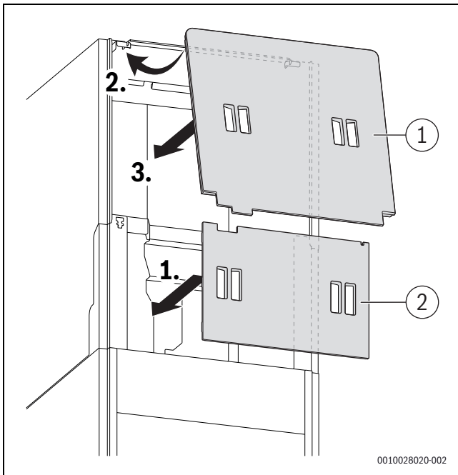
Bild 101 Wärmedämmung an der Rückseite anbringen (Zubehör SF 13)
