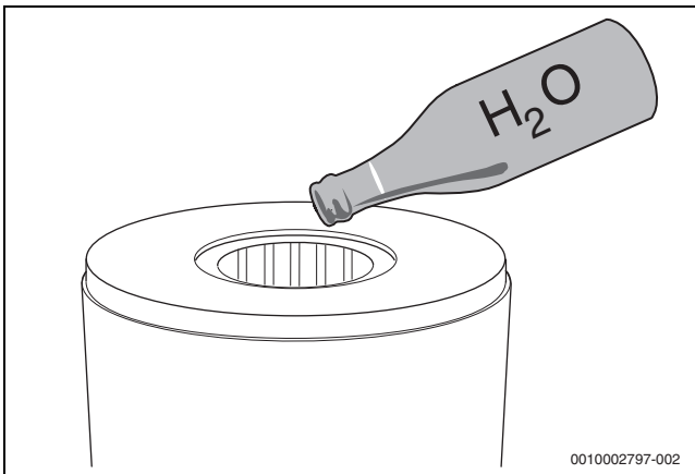
Bild 137 Wärmeblock mit Wasser spülen
