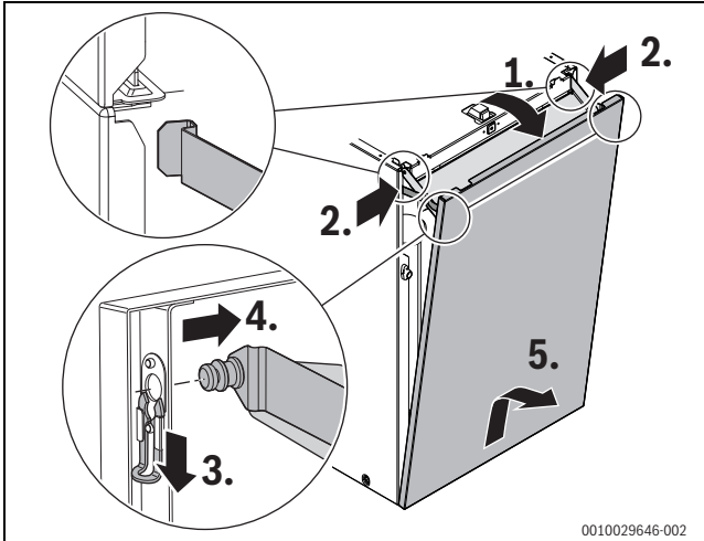
Bild 165 Vorderteil der Speicherverkleidung abnehmen und sicher abstellen
