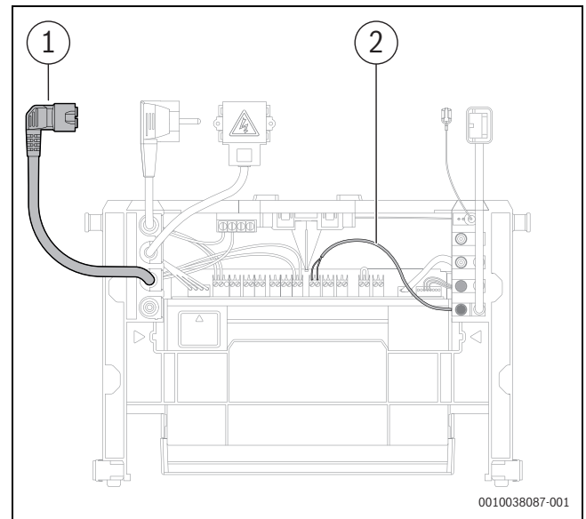
Bild 88 Steckplatz für Schichtladepumpe und Anschluss des Warmwasserspeicher-Temperaturfühlers
