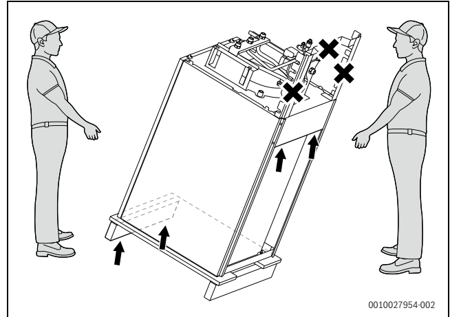
Bild 52 Transport des Speichers
