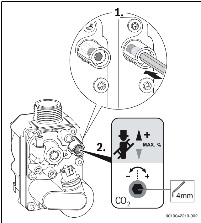
Bild 112 CO 2 /O 2 -Gehalt bei maximaler Nennwärmeleistung einstellen
