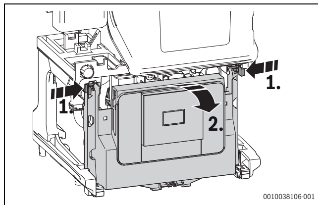
Bild 63 Steuergerät herunterklappen
