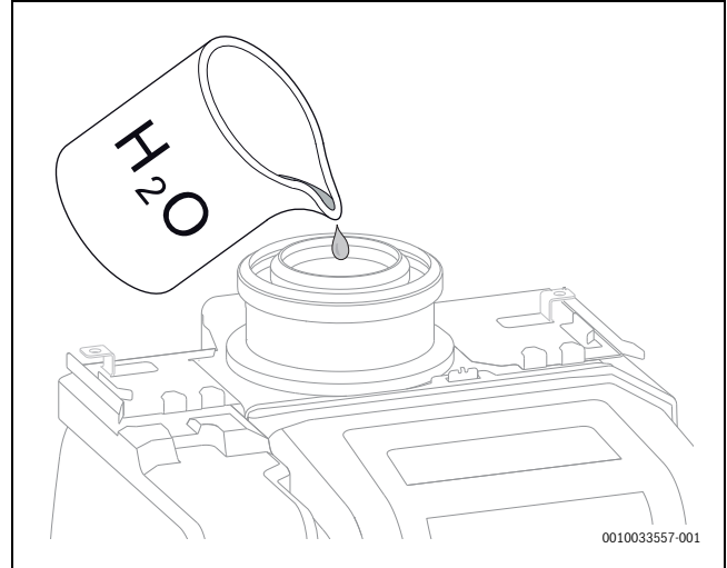
Bild 76 Kondensatsiphon mit Wasser füllen
