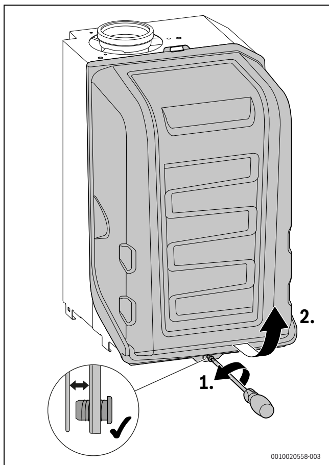
Bild 82 Brennerhaube abnehmen
