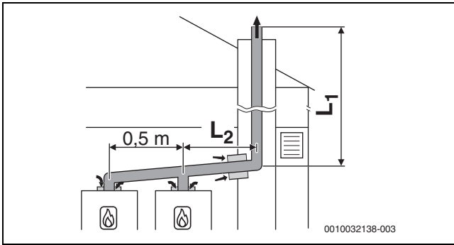
Bild 46 Kaskade mit 2 Geräten: Starre Abgasführung im Schacht nach B 53p mit raumluftabhängiger Luftzufuhr am Gerät
