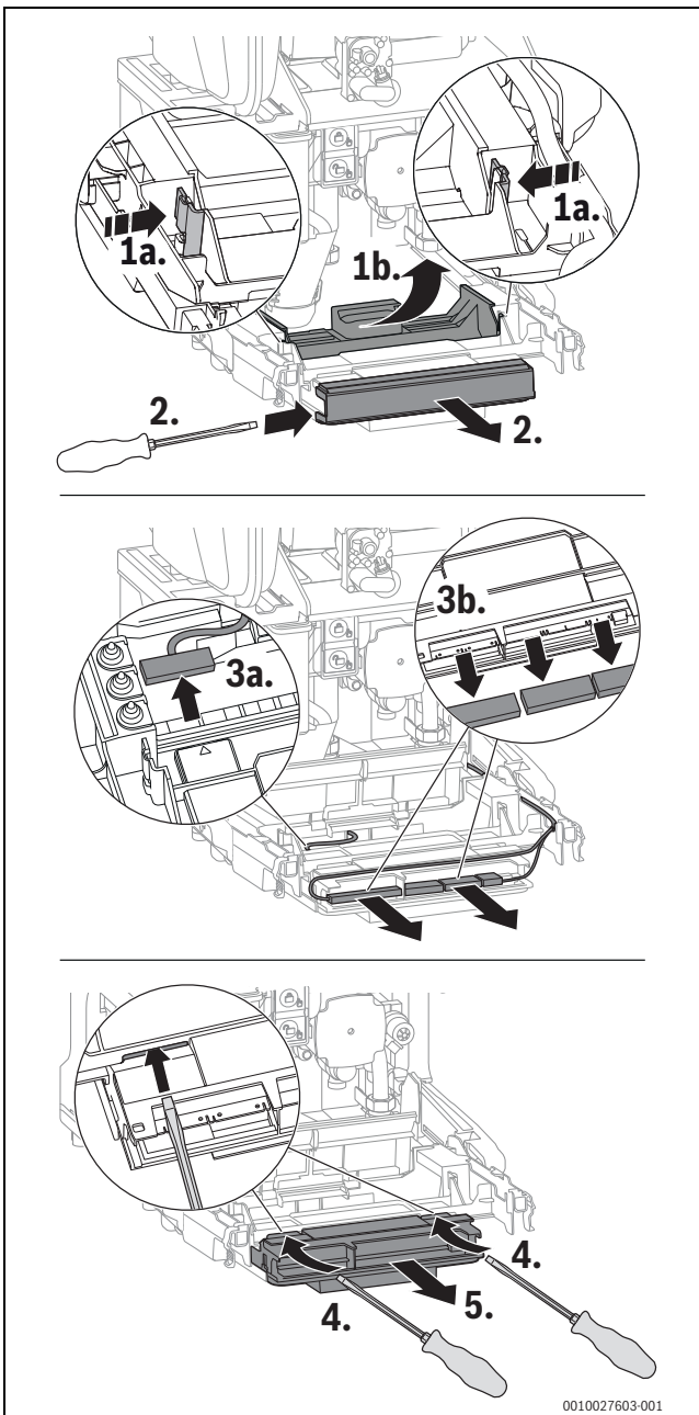
Bild 152 Steuergerät herausnehmen
