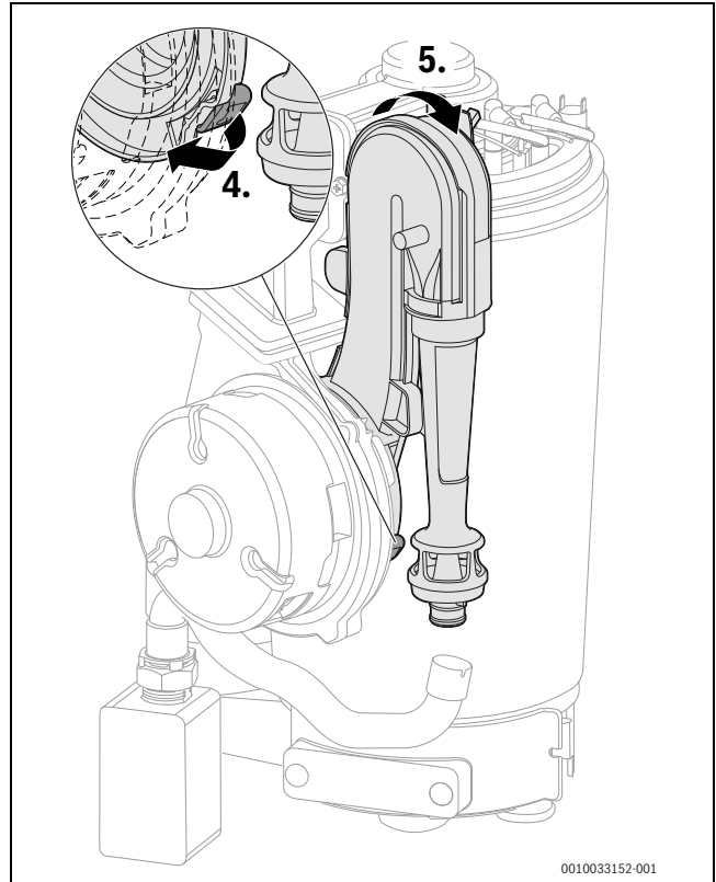
Bild 124 Venturirohr abnehmen
