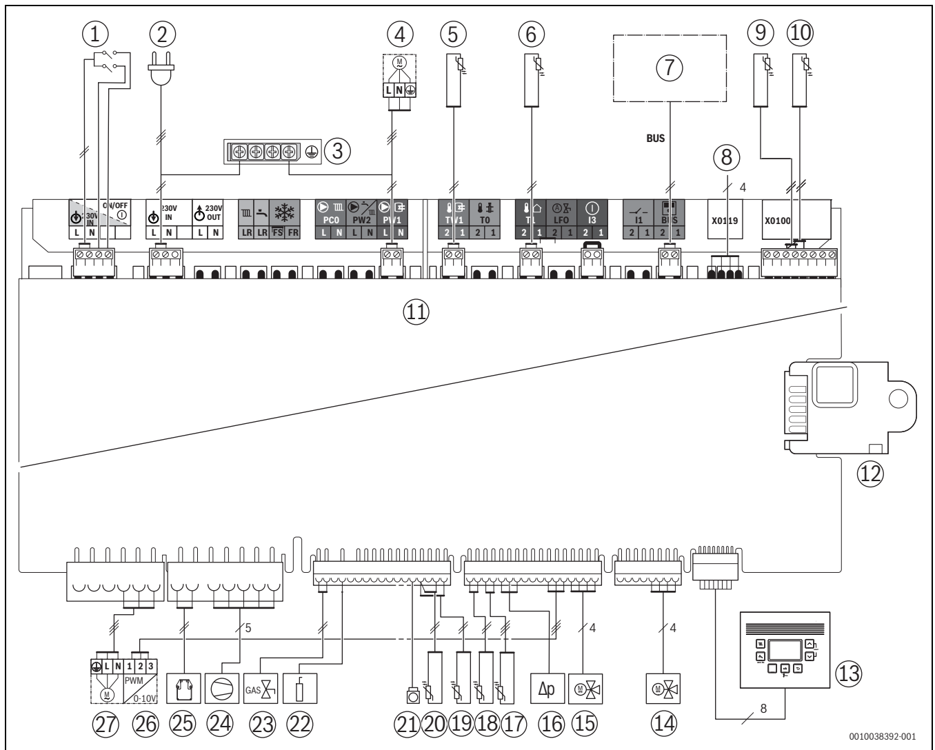
Bild 167 Elektrische Verdrahtung
