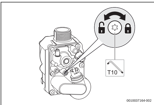
Bild 110 Gas-Anschlussdruck messen
