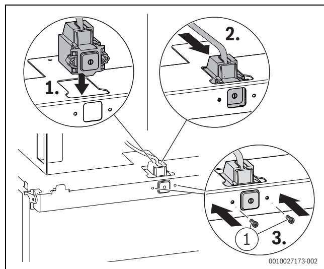
Bild 84 Schalter Ein/Aus befestigen
