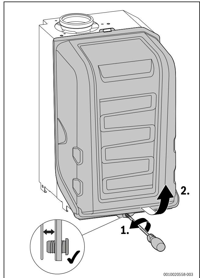
Bild 109 Brennerhaube abnehmen
