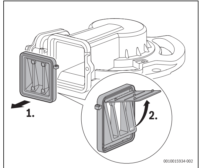
Bild 128 Rückströmsicherung in der Mischeinrichtung
