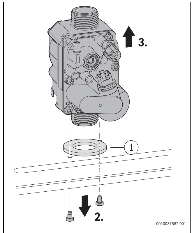
Bild 147 Gasarmatur ausbauen
