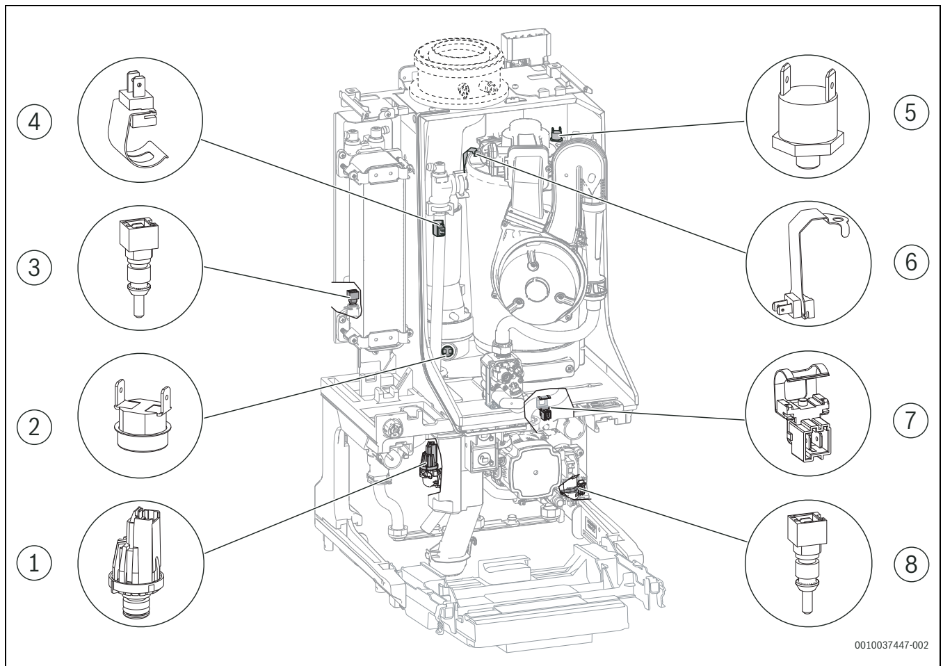
Bild 5 Fühler und Sensoren im Gerät
