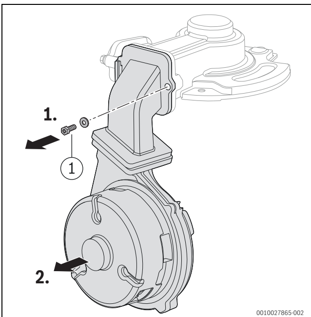
Bild 127 Mischeinrichtung und Gebläse ausbauen
