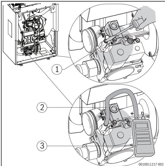
Bild 39 Gas-Anschlussdruck messen
