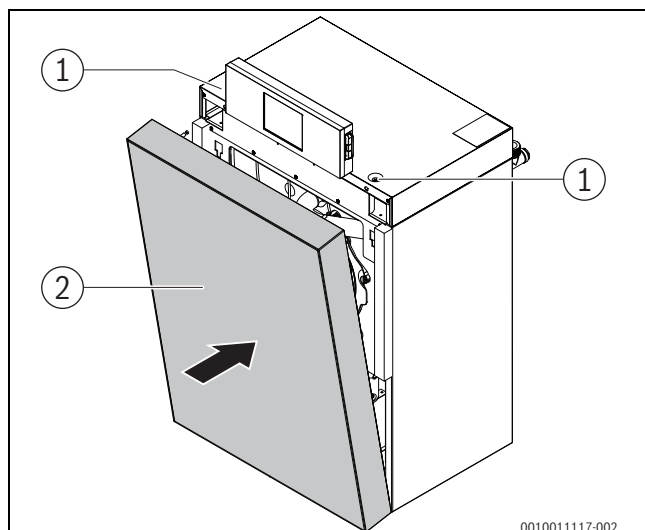
Bild 44 Kesselvorderwand montieren
