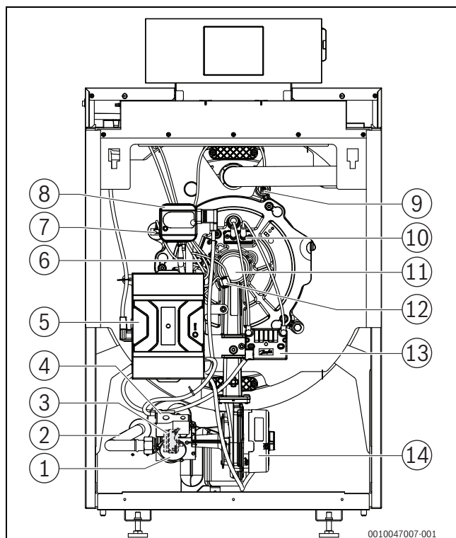
Bild 80 Vorderansicht
