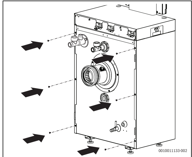
Bild 67 Seitenwände befestigen
