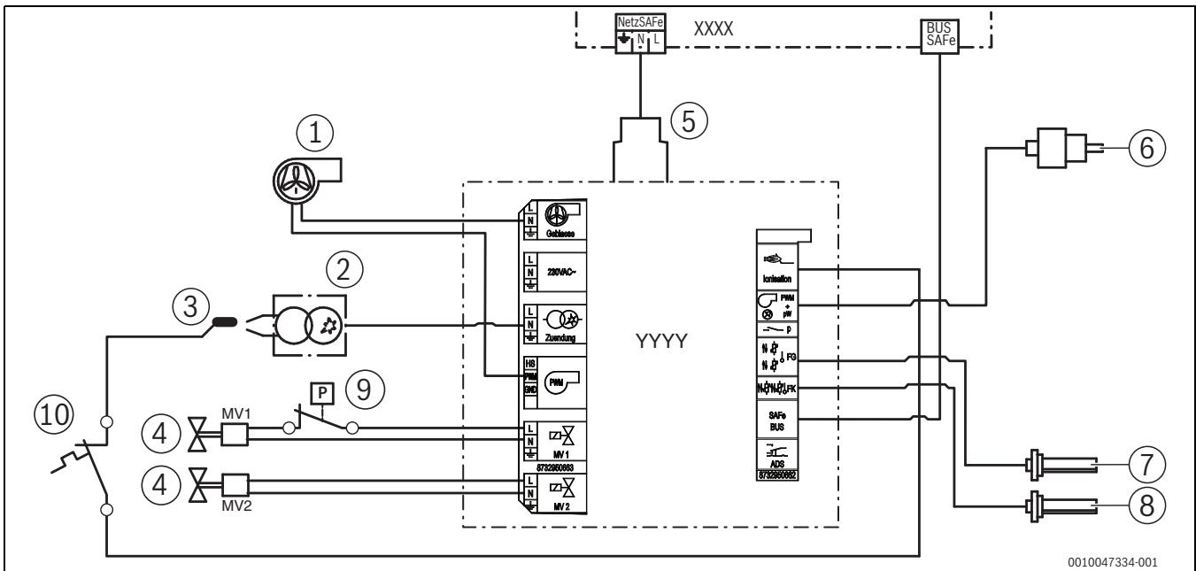
Bild 79 Anschlussplan Feuerungsautomat
