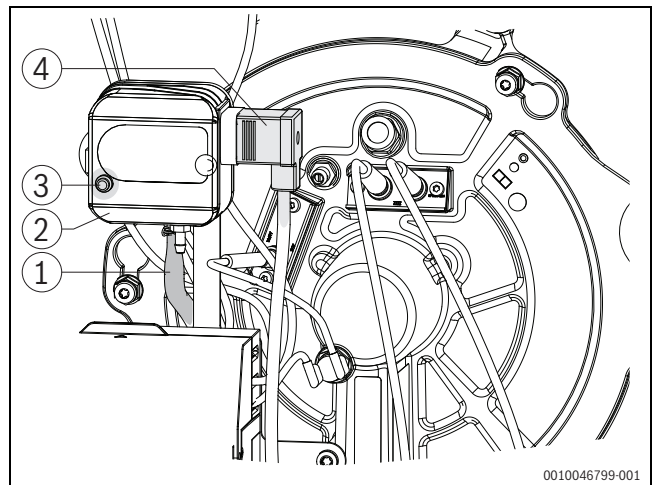
Bild 71 Feuerraum-Druckwächter
