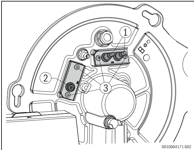
Bild 58 Elektrodenposition
