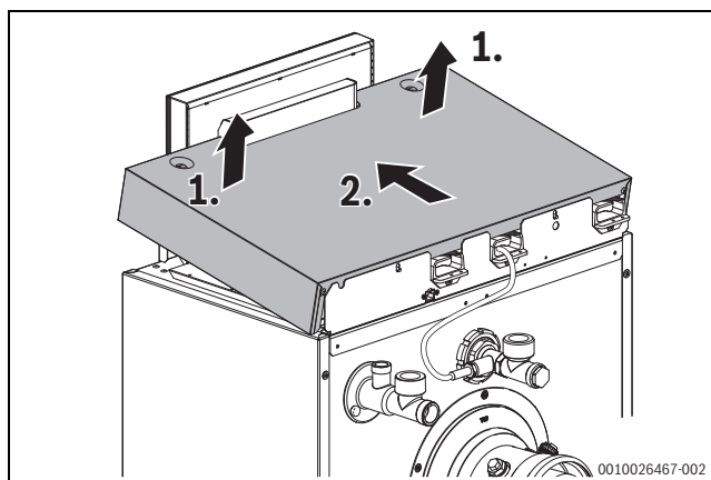
Bild 19 Kesselhaube abnehmen
