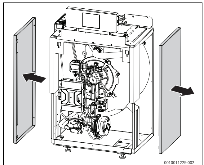
Bild 64 Seitenwände abnehmen
