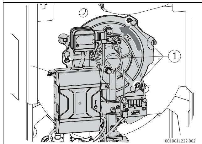
Bild 53 Befestigungsmuttern lösen
