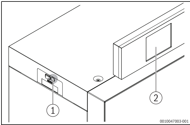
Bild 77 Geräteversicherung am Regelgerät IMC120 mit Bedienfeld BC400
