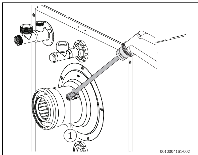
Bild 41 CO/CO 2 /O 2 -Gehalt messen
