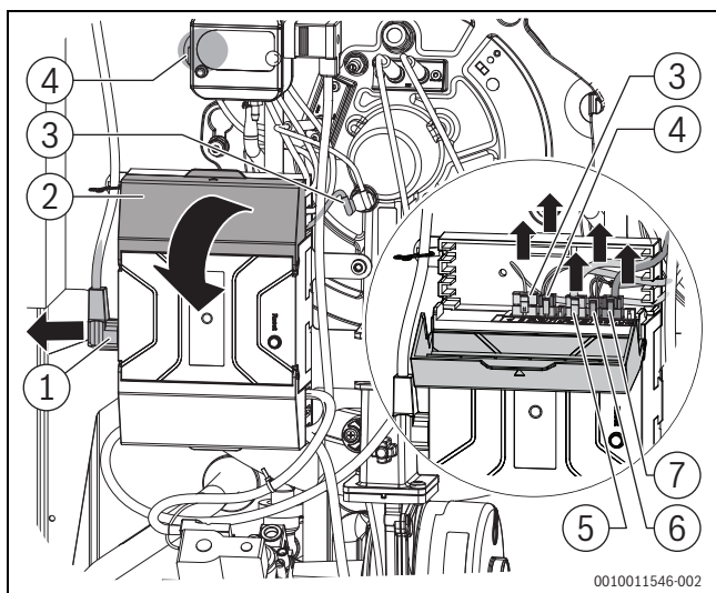
Bild 50 Steckverbinder lösen
