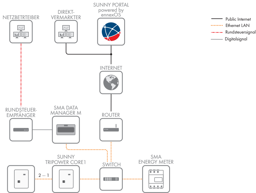
Abbildung 5: Aufbau Anlagenkommunikation
