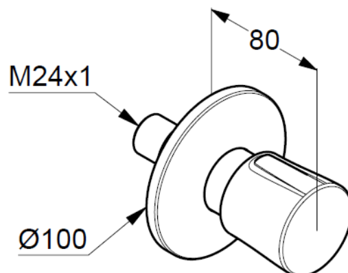
Maßzeichnung/ Dimensional drawing
