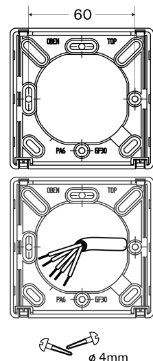
DE Unterputzdose EN Flush-mounting box
