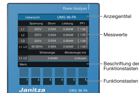
Abb. Standardanzeige UMG 96-PA / MID+ - Messwertanzeige „Übersicht“
