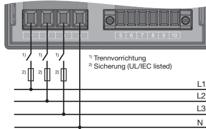
Abb. Anschlussvariante „Direkte Spannungsmessung in einem Dreiphasen-Vierleitersystem“
