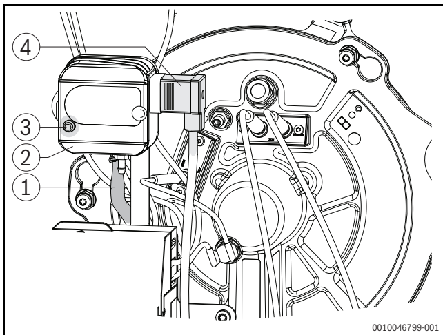
Bild 71 Feuerraum-Druckwächter
