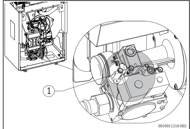
Bild 32 Gasleitung entlüften
