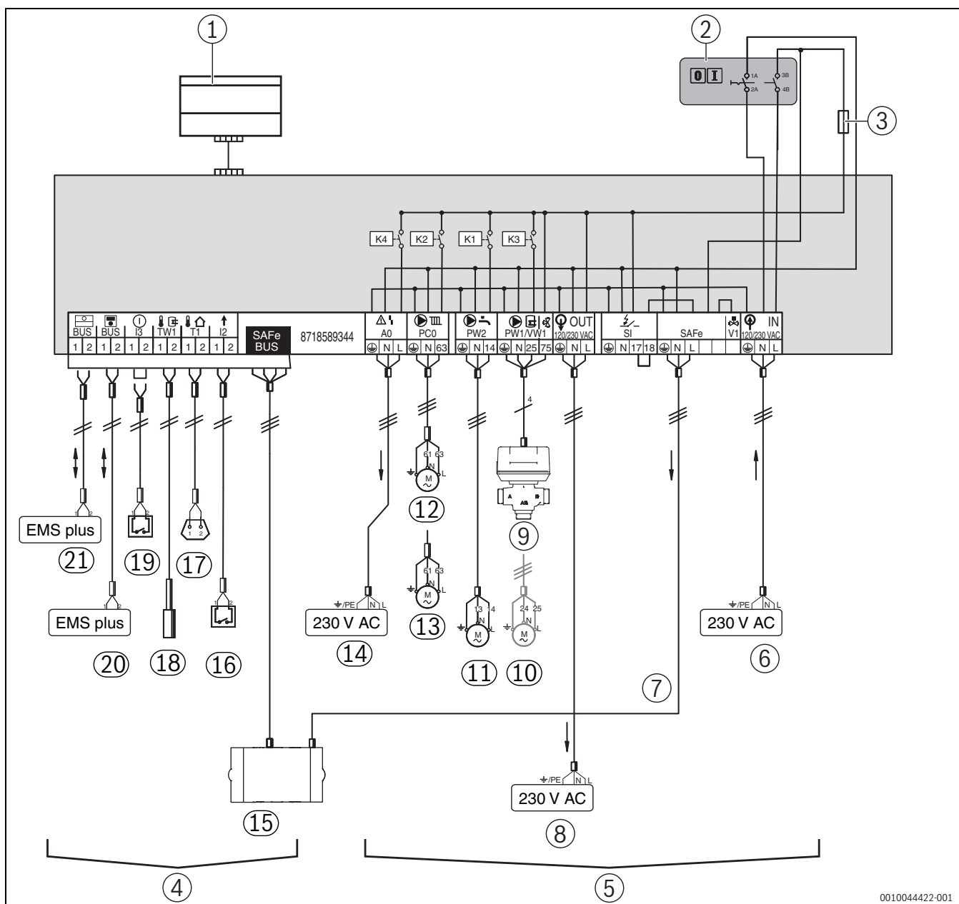
Bild 76 Anschlussplan Regelgerät IMX35
