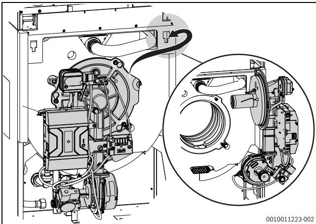
Bild 54 Brenner in Wartungsposition
