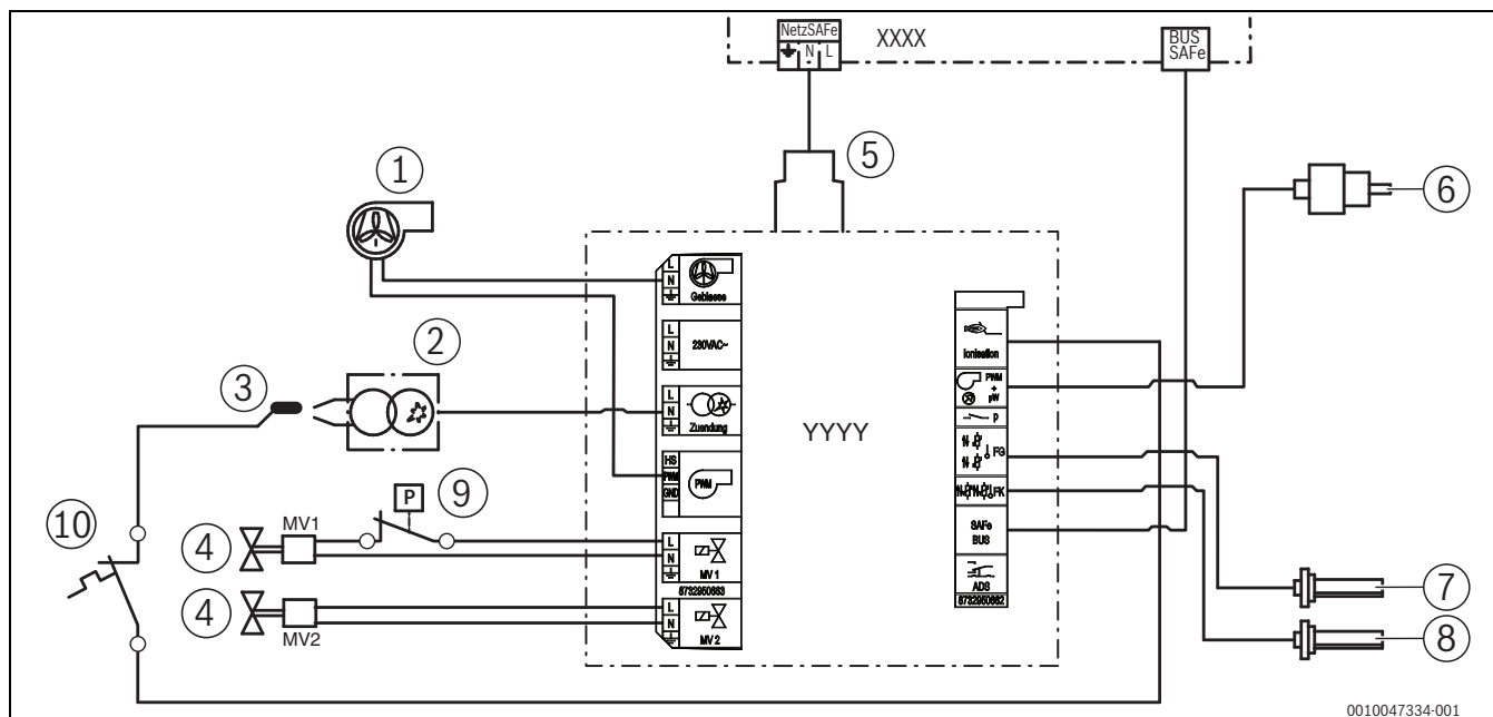
Bild 79 Anschlussplan Feuerungsautomat (bei manchen Modellen)
