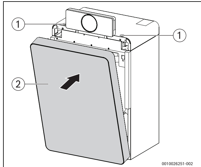
Bild 44 Kesselvorderwand montieren
