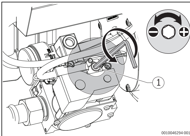
Bild 40 Einstellung Teillast
