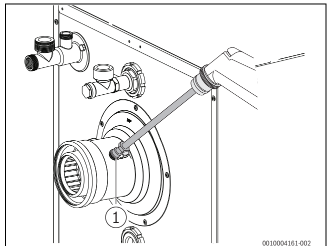
Bild 43 Messwerte aufnehmen
