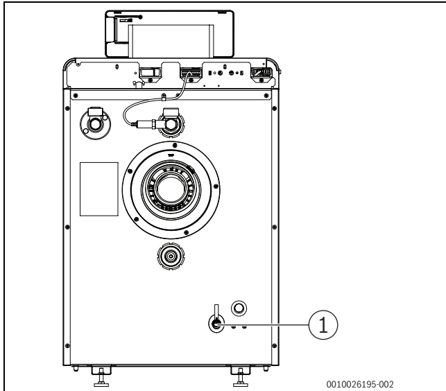
Bild 14 Kondensatschlauch montieren
