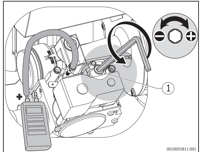
Bild 42 Einstellung Teillast
