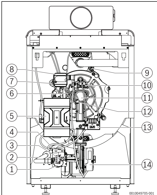
Bild 81 Vorderansicht
