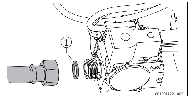
Bild 52 Gasrohr abnehmen
