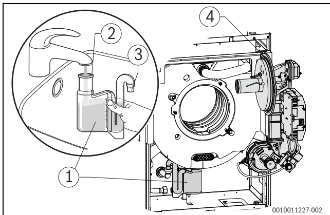
Bild 60 Siphon reinigen
