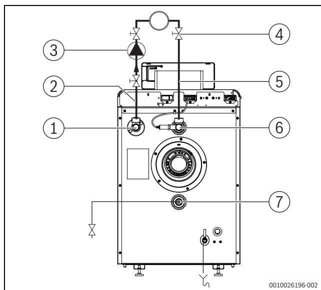
Bild 15 Anschlussschema Hydraulik
