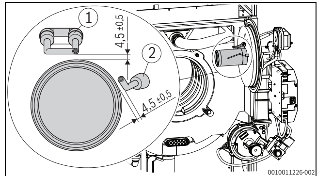
Bild 59 Abstände Elektroden
