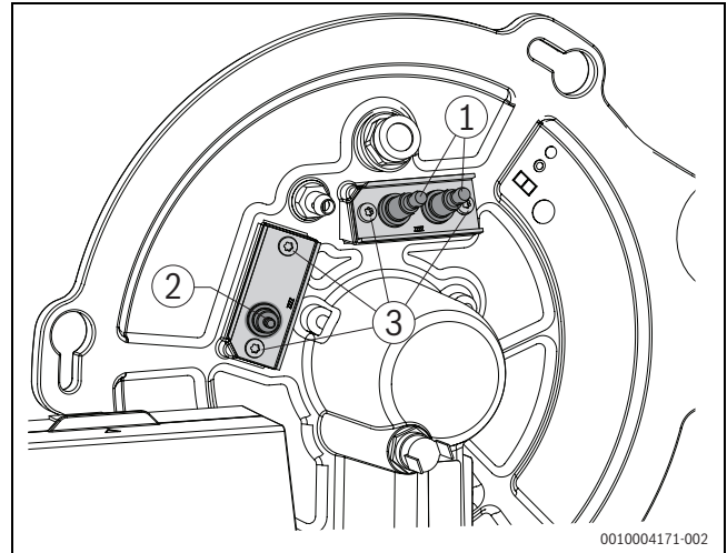
Bild 58 Elektrodenposition
