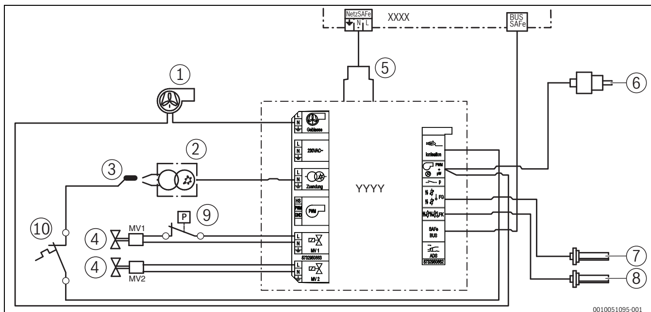
Bild 80 Anschlussplan Feuerungsautomat (bei manchen Modellen)
