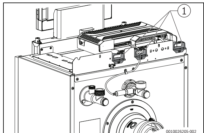
Bild 21 Kabel verlegen
