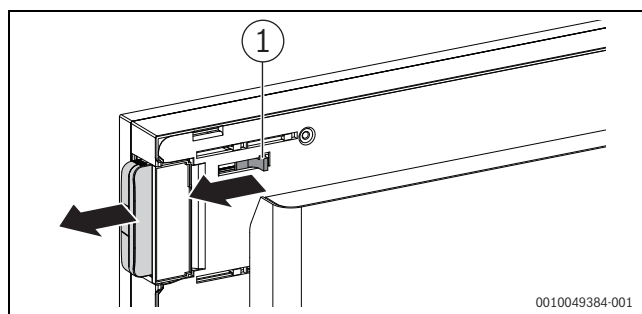
Bild 35 Kommunikationsmodul demontieren
