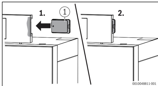
Bild 34 Kommunikationsmodul montieren
