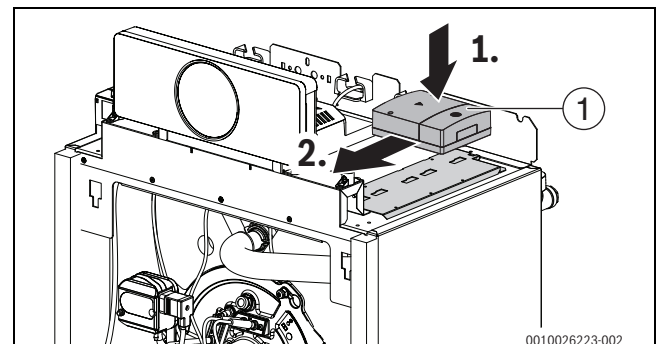
Bild 26 Funktionsmodule einstecken
