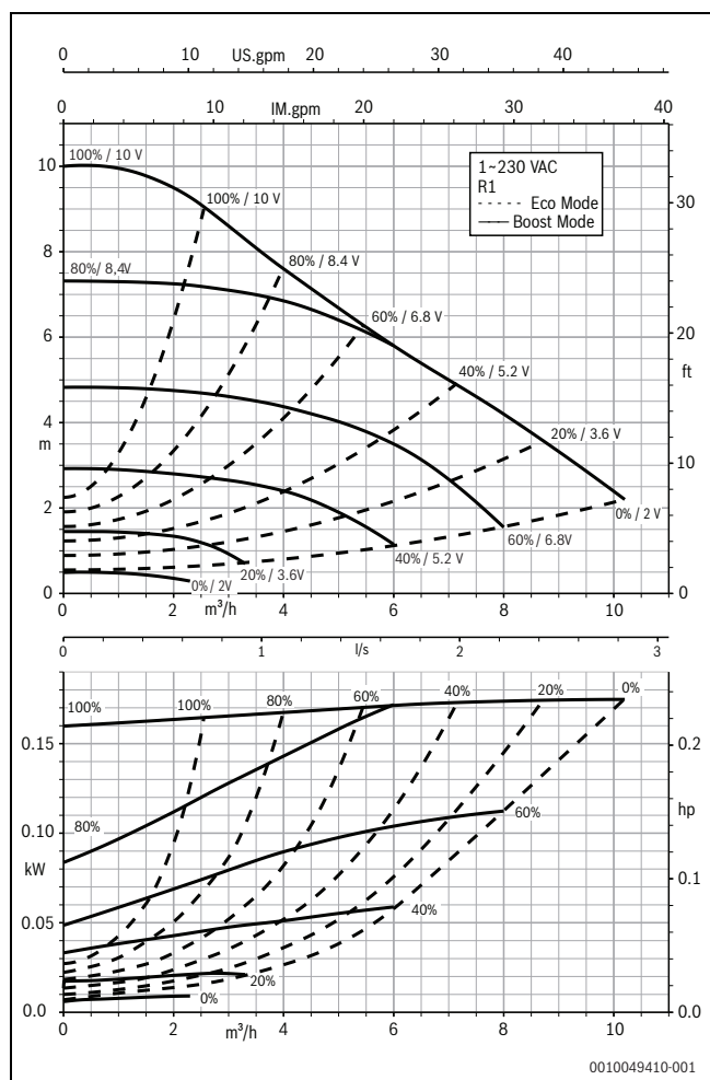
Fig. 10 Pumpekurver Calio 25-100
