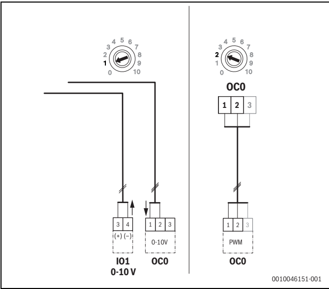
Fig. 5 EM100/ OCO 1-2 udgang kontrollsignal pumpe (nominel værdi 0-10 V/PWM)
