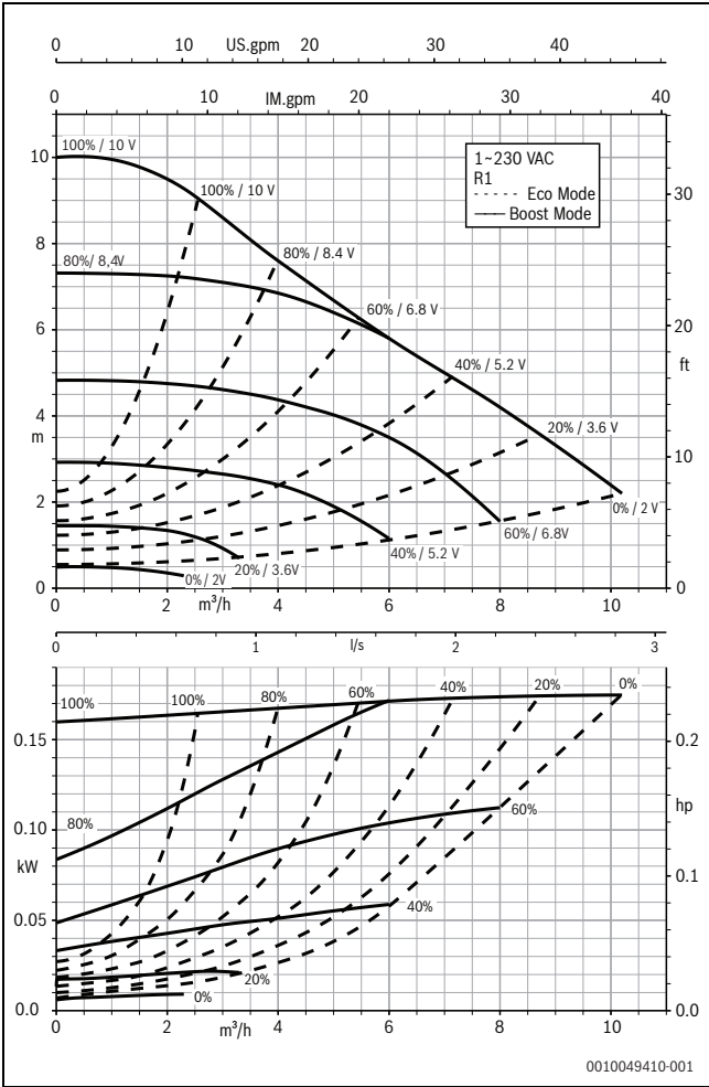
Bild 10 Pumpenkennlinien Calio 25-100
