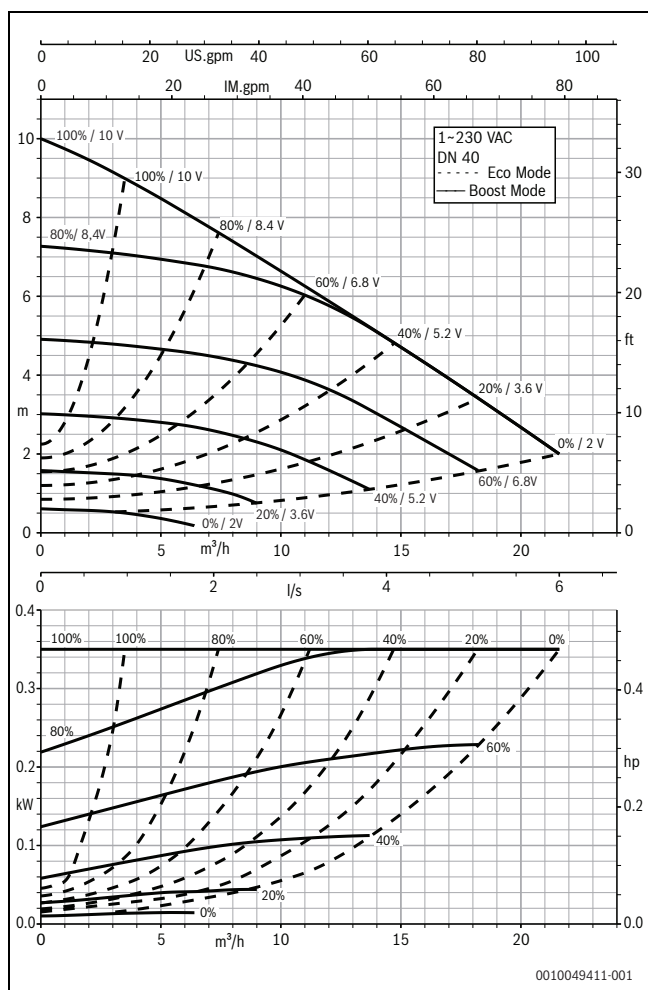
Afb. 11 Opvoercharacteristieken Calio 40-100
