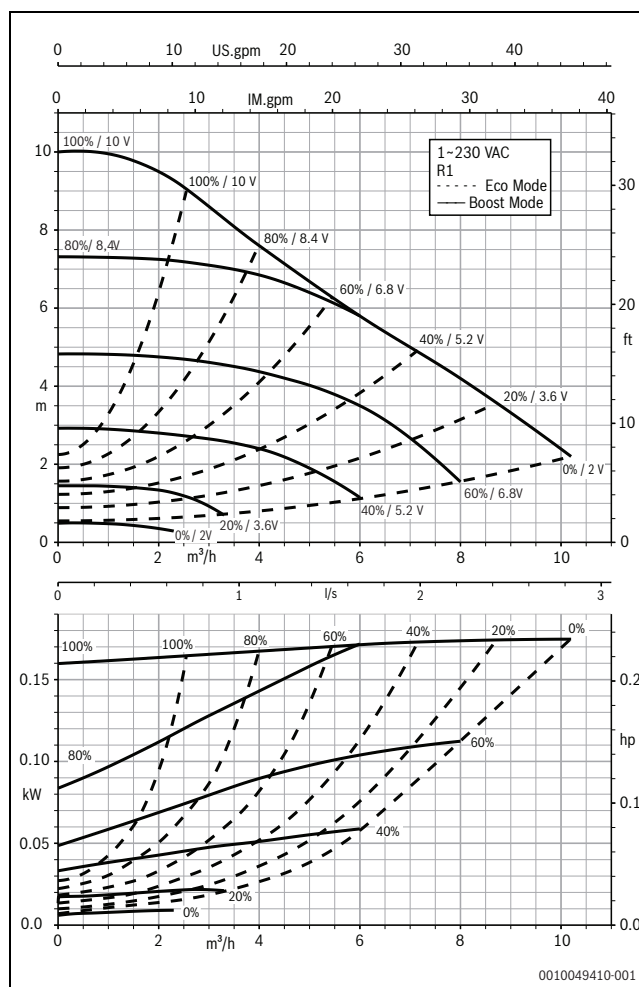
Afb. 10 Opvoercharacteristieken Calio 25-100
