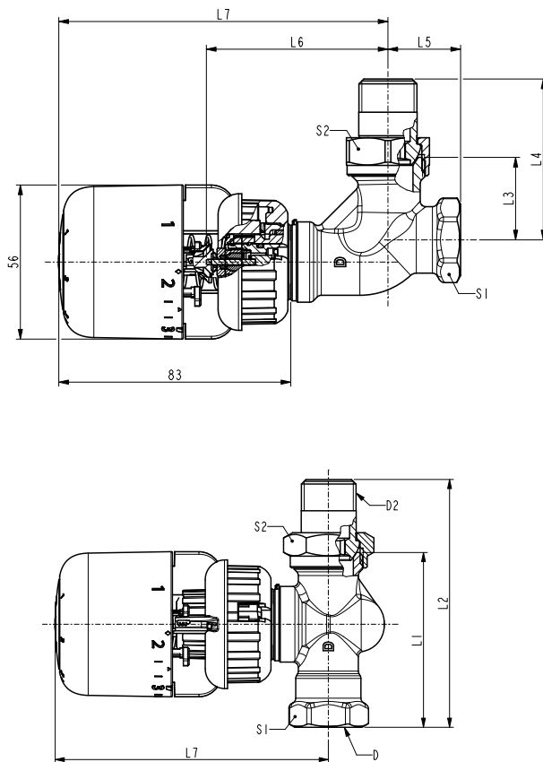
RA-DV DN 20 Durchgangs- und Eckventil/Fühler Danfoss Aero®
