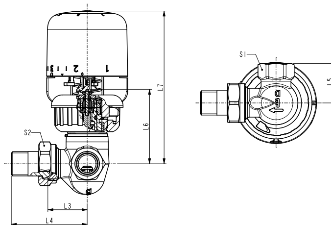
RA-DV Durchgangsventil/ Danfoss Aero® Fühler
