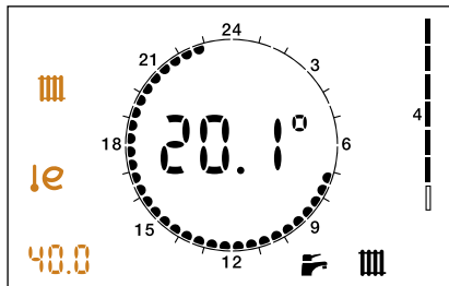
Rücklauftemperatur Primärkreislauf Grenz-/Einstellwert im Heizbetrieb (**) (SATK2210. - SATK2220.)
