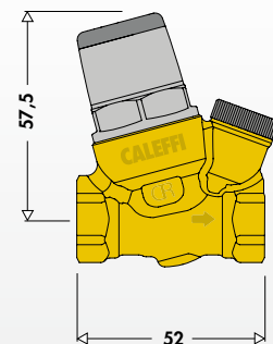
MIKRO-Schrägsitz- Druckminderer 3/8"
