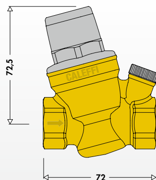
Schrägsitz-Druckminderer 1/2"
