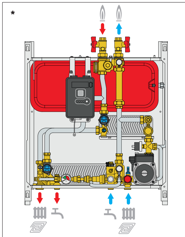
NB: Die Ventile laut Abbildung installieren
