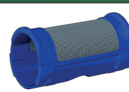
Vorreinigungssieb Maschenweite Ø = 0,30 mm
