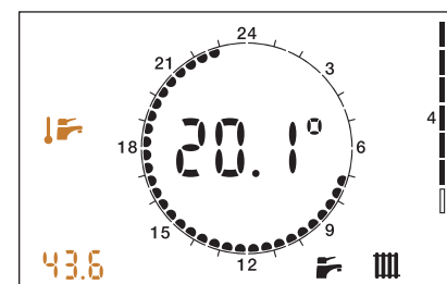
Temperatur des Fühlers für warmes Brauchwasser
