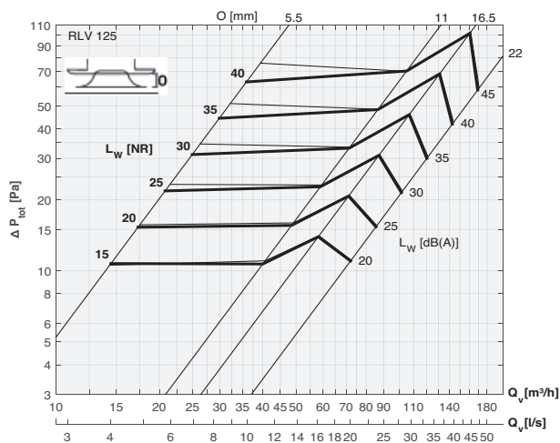
Druck-Volumenstromkennlinie Abluft
