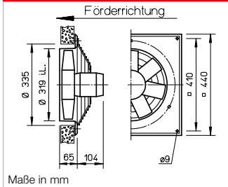
Maße HQ EC 315
