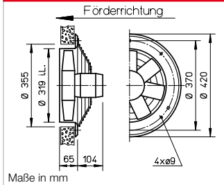
Maße HW EC 315
