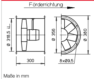
Maße HRF EC 315
