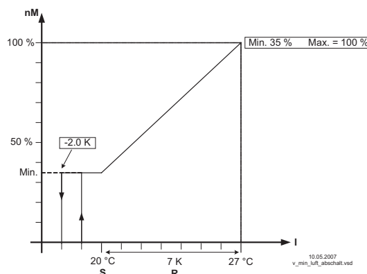
Mindestluftabschaltung (idealisiertes Prinzipschaubild)
