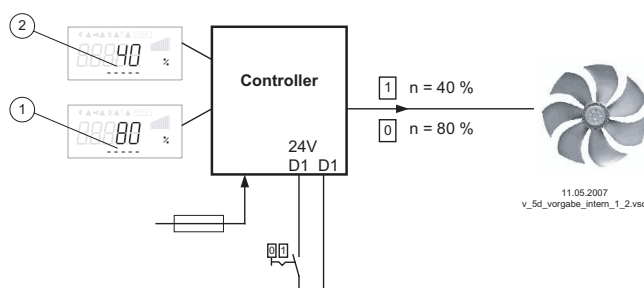
1 Einstellung "Vorgabe Intern1" (je nach Geräteart in: %, Hz, rpm)
