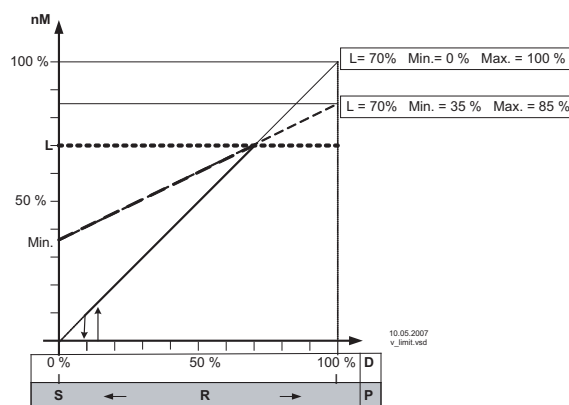
Limit (idealisiertes Prinzipschaubild)
