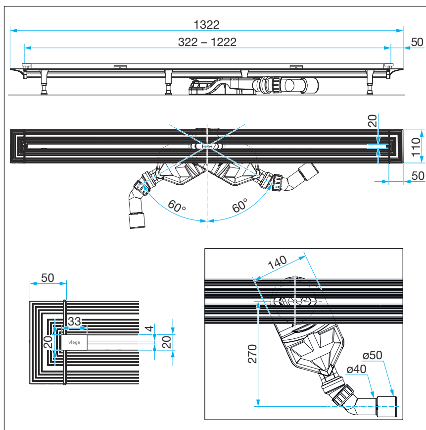
Abb. 13: Abmessungen Grundkörper Basismodell
