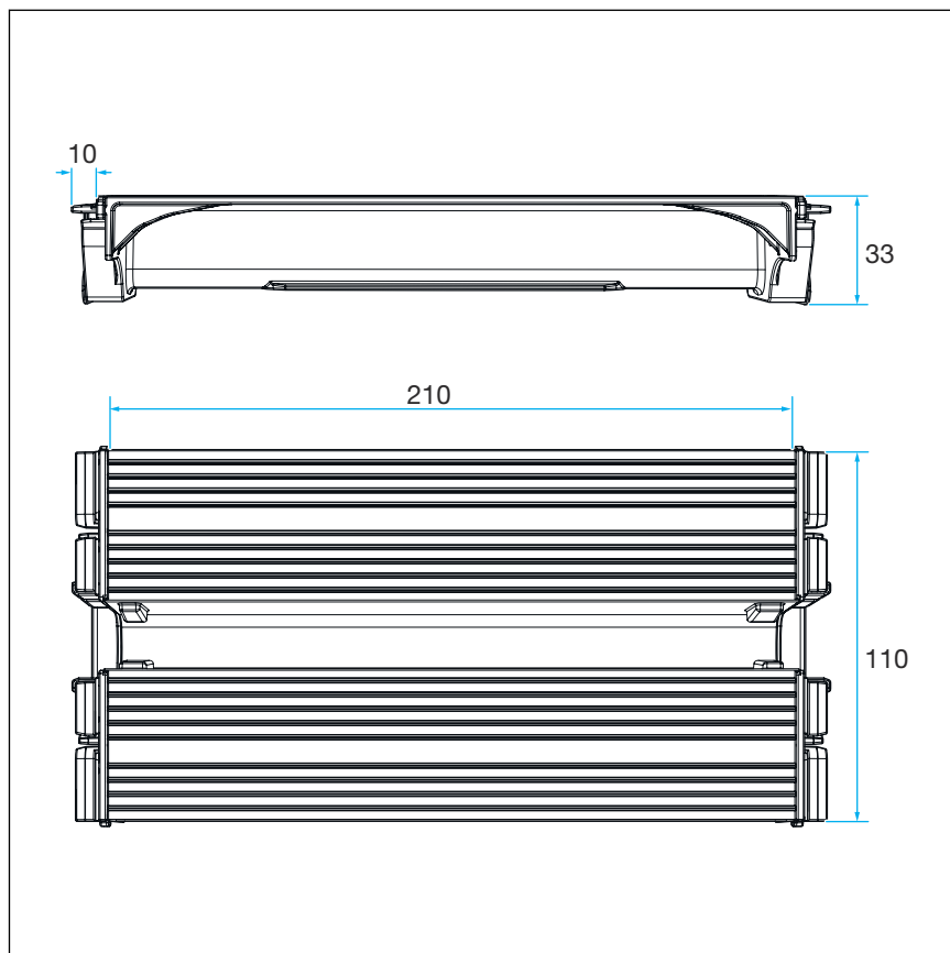
Abb. 14: Abmessungen Verbindungsstück
