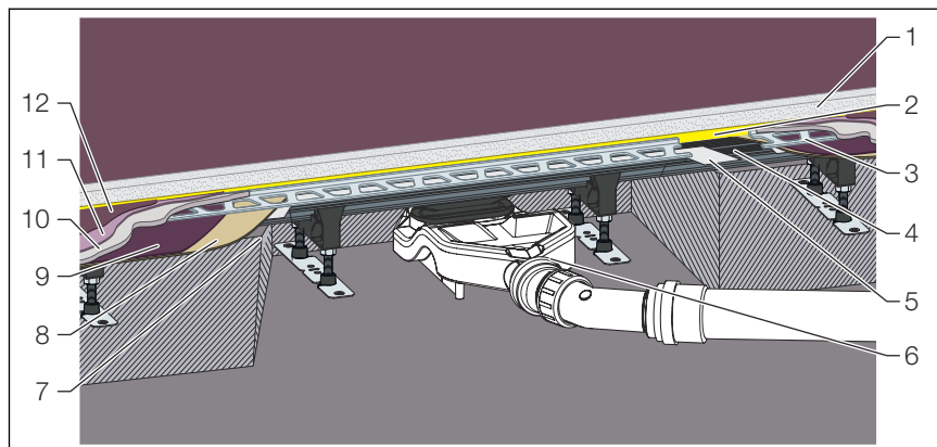
Abb. 20: Schichtaufbau der Verlaufsbeschichtung
