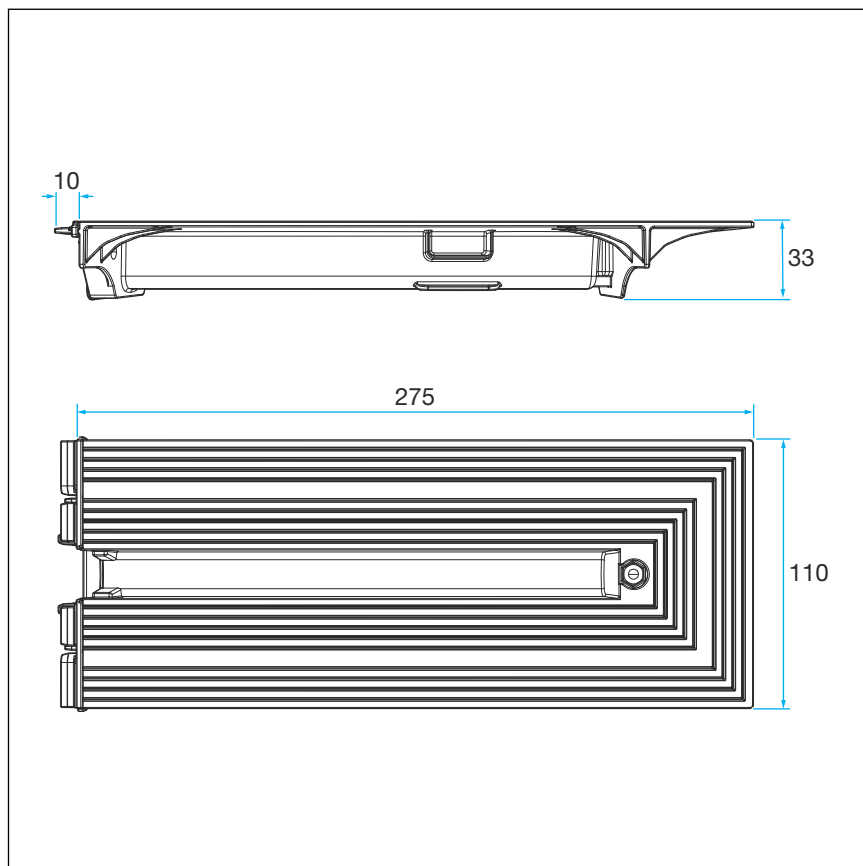
Abb. 15: Abmessungen Endverschlussstück
