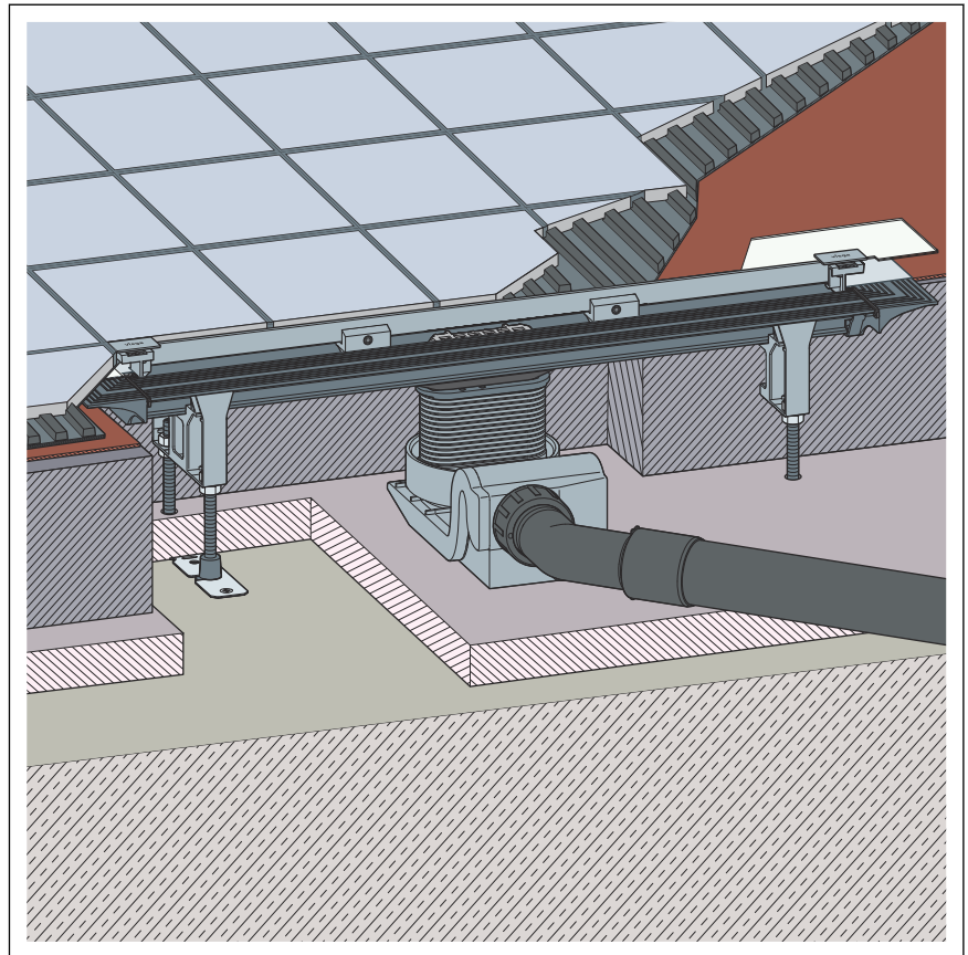
Abb. 9: Schema einer Verbundabdichtung
