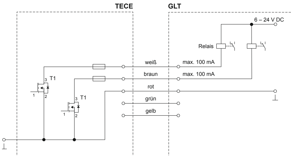
Anschluss an GLT mit externem Netzteil (B)
