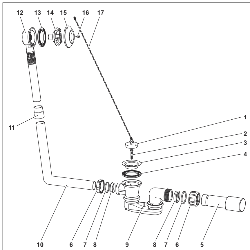
Abb. 1: Bauteilübersicht
