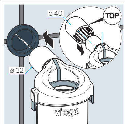
Abb. 2: Montagemaße
