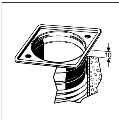
Abb. 4: Minimale Einbauhöhe
