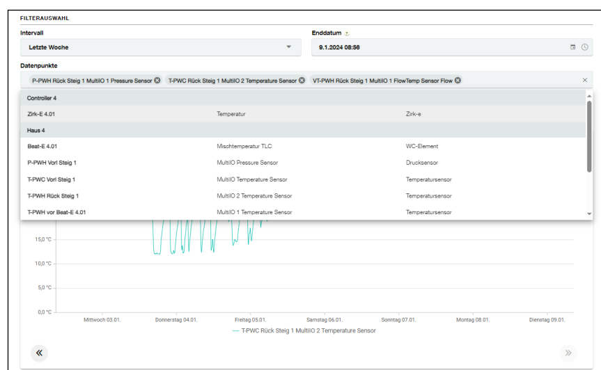
Abb. 3: Filterauswahl
