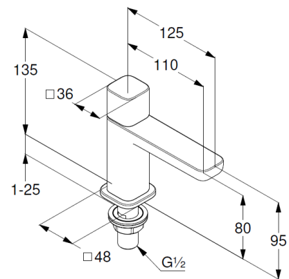
Maßzeichnung/ Dimensional drawing
